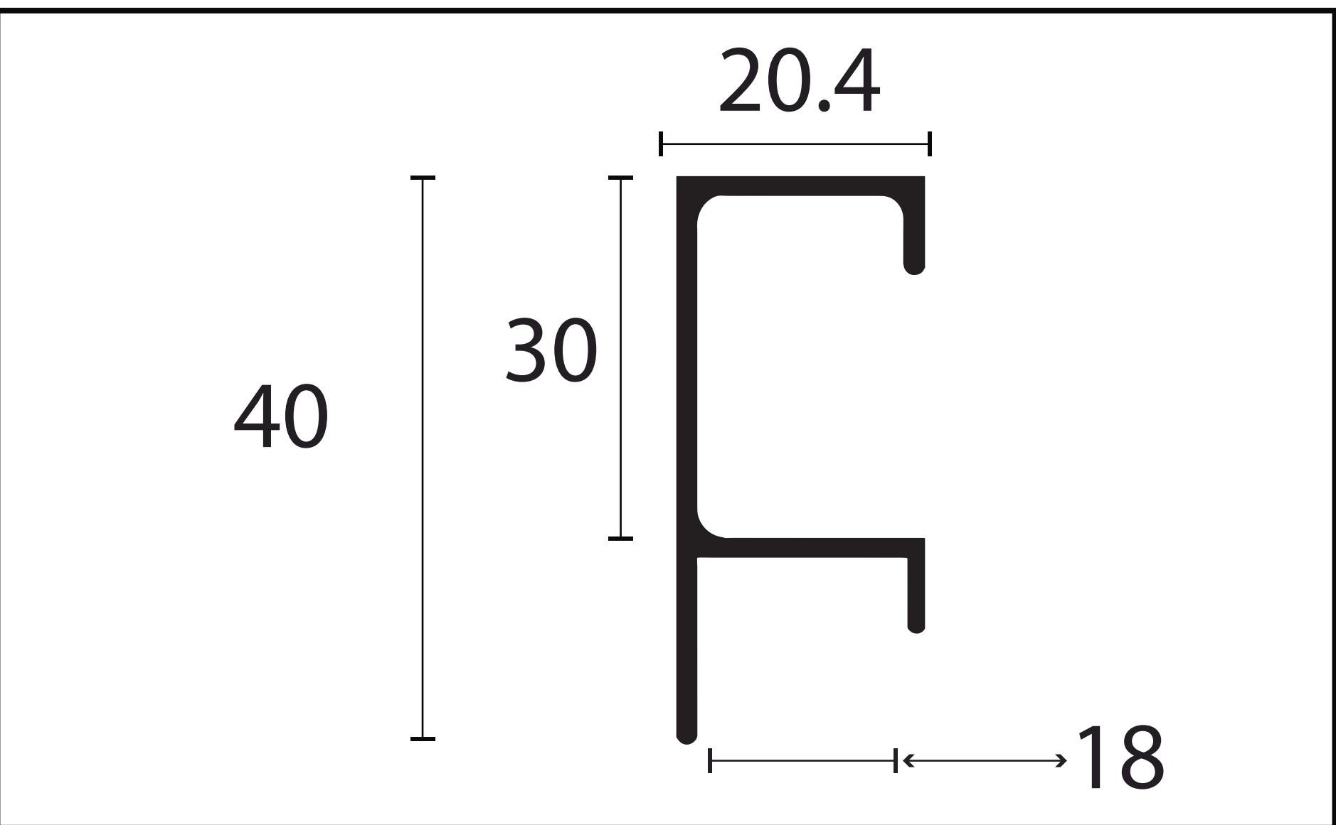
PUXADOR GAP - 9522
