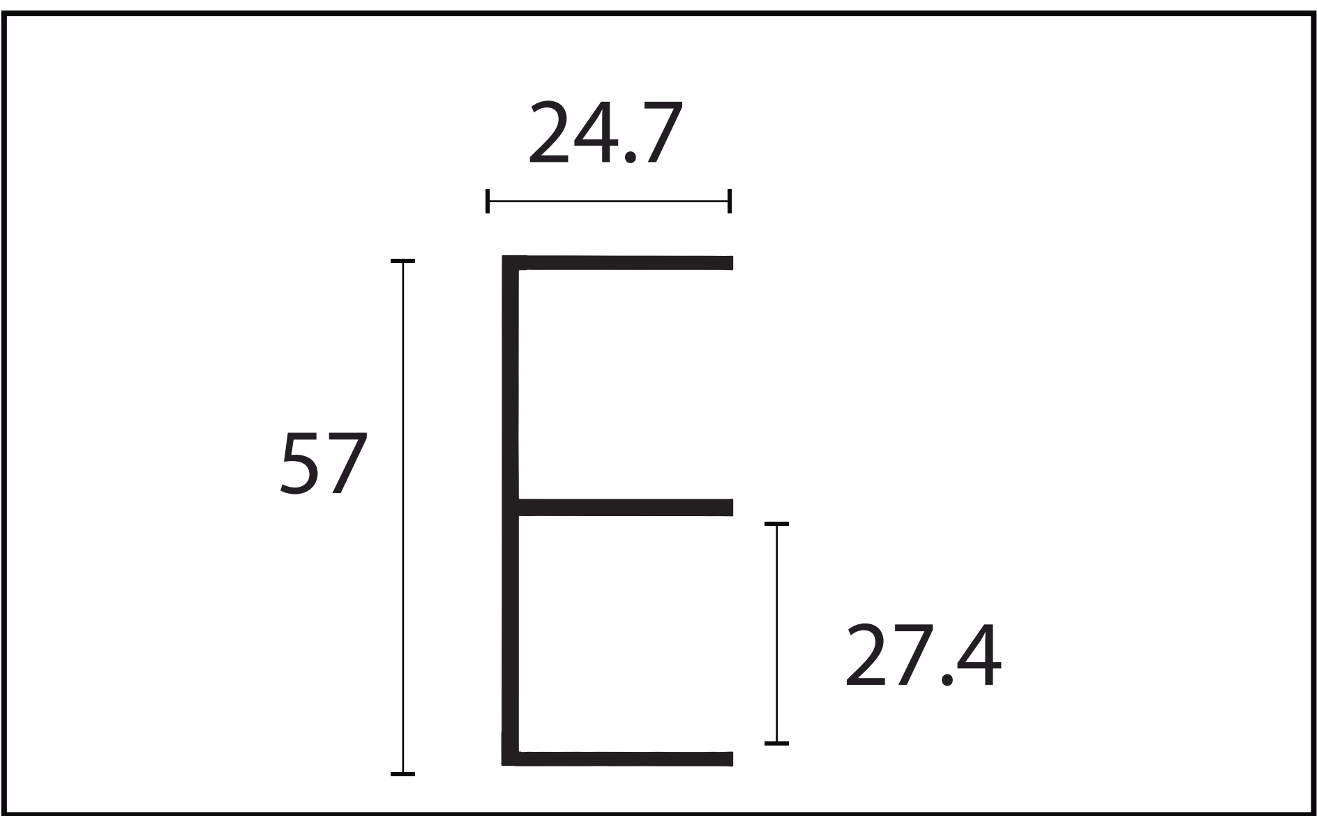
TRILHO GAP - 9013 P/E
