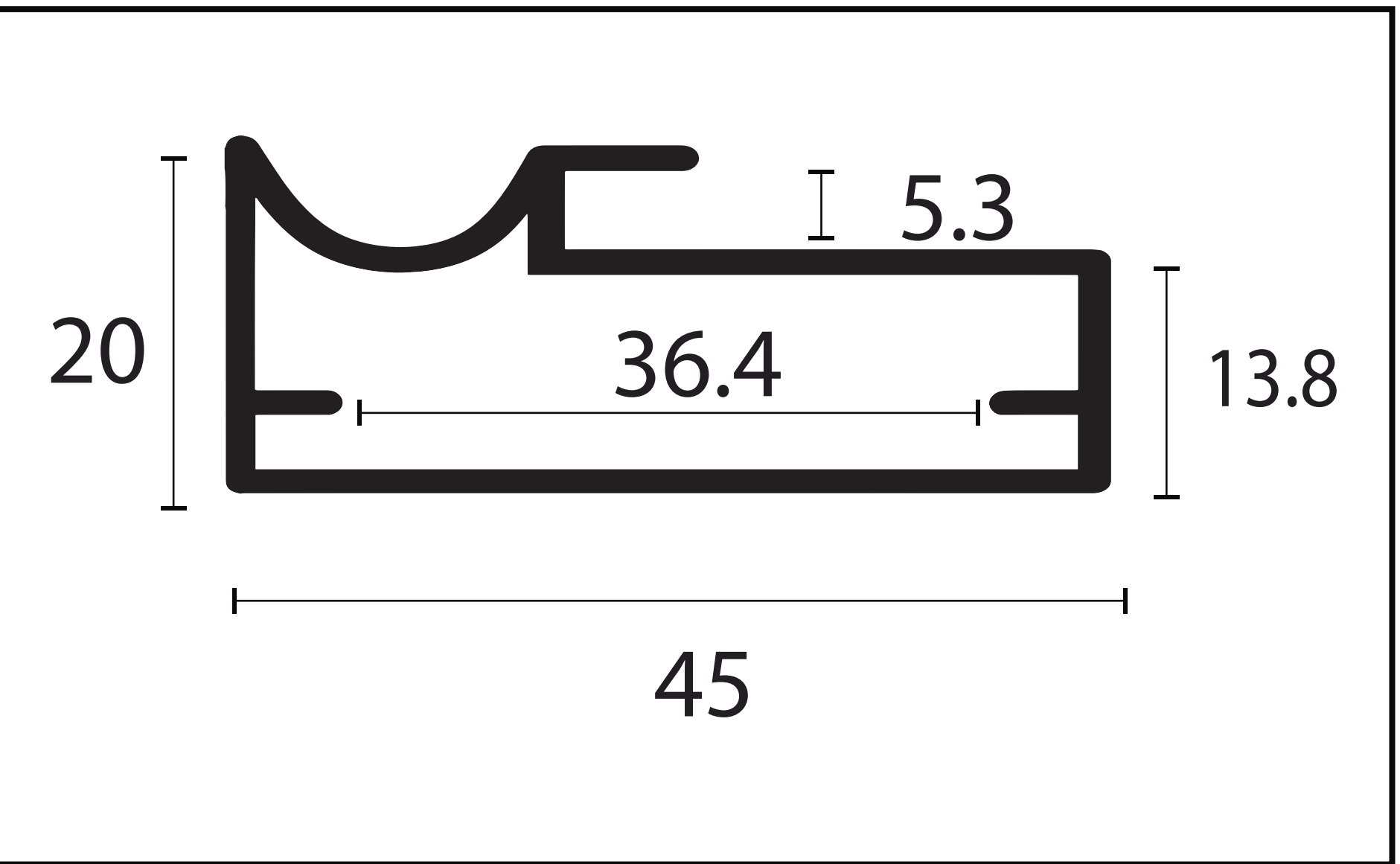
MONTANTE GAP - 8888
