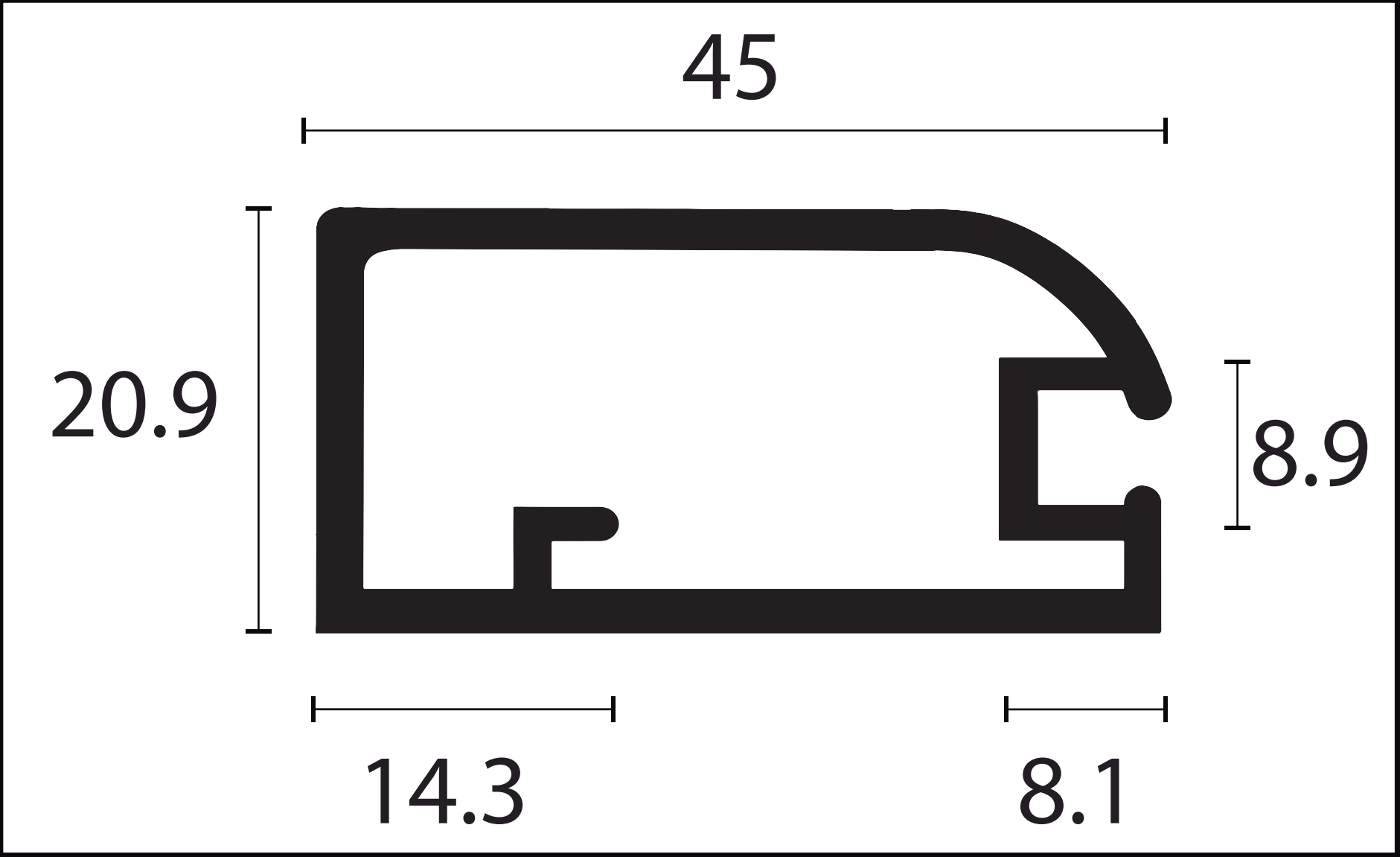
MONTANTE GAP - 1491
