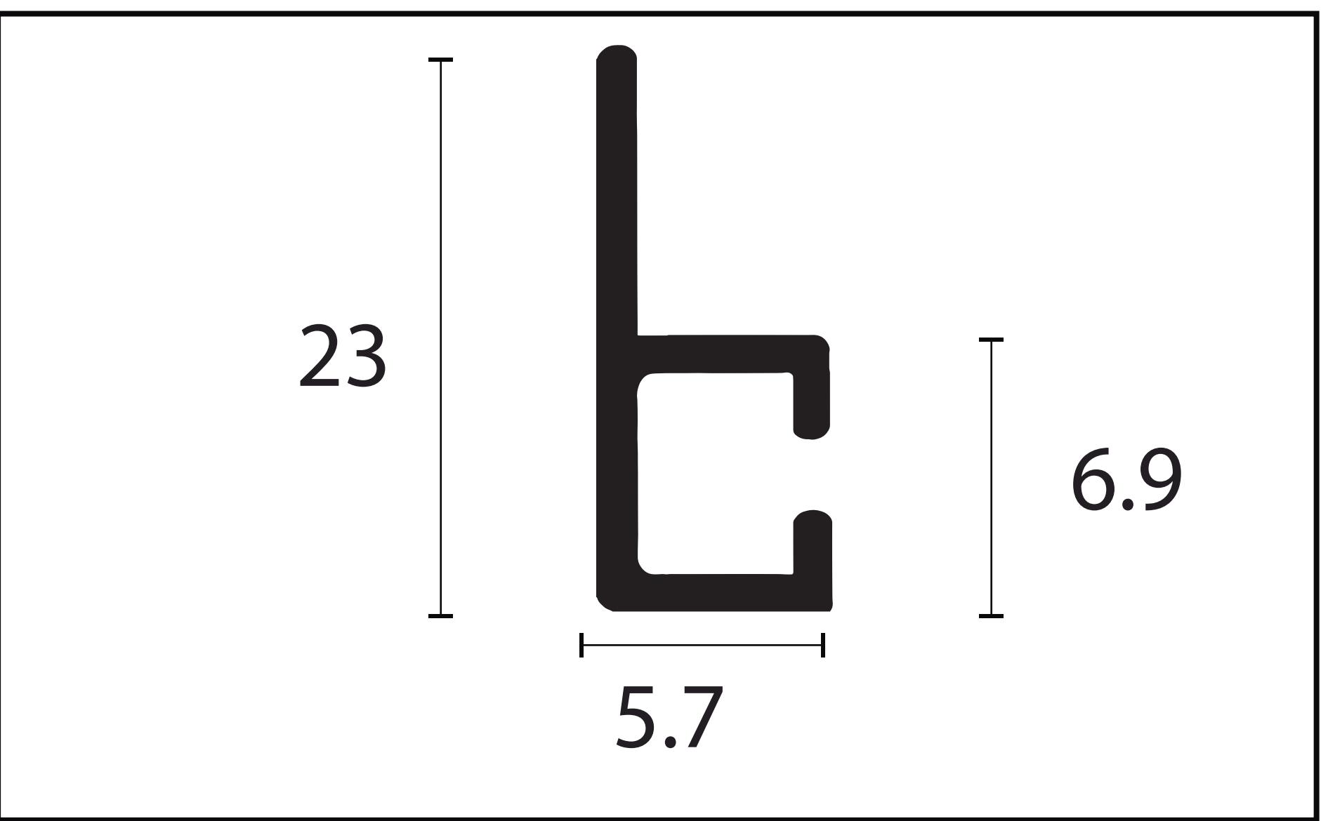
TRILHO GAP - 1818
