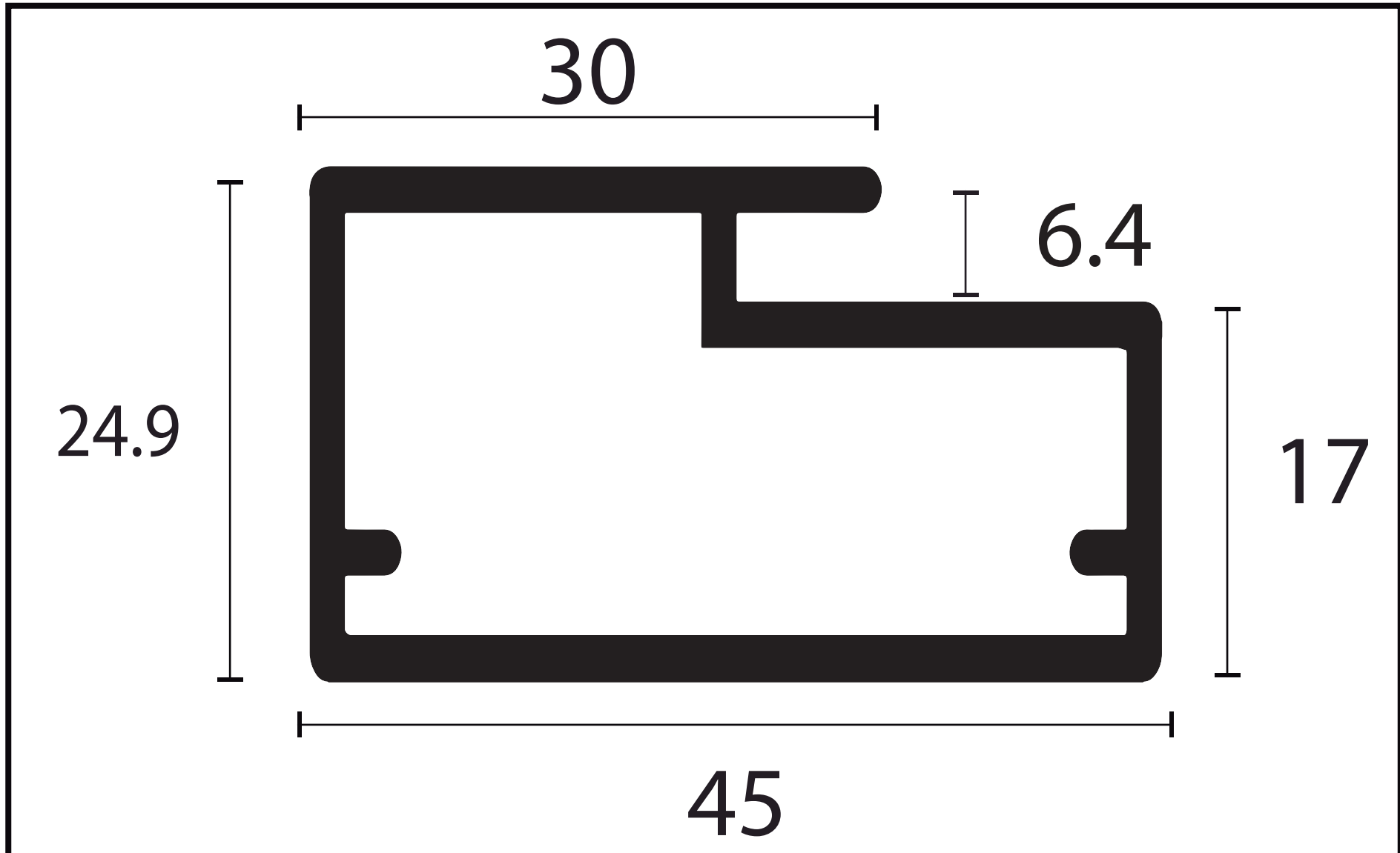
MONTANTE GAP - 997
