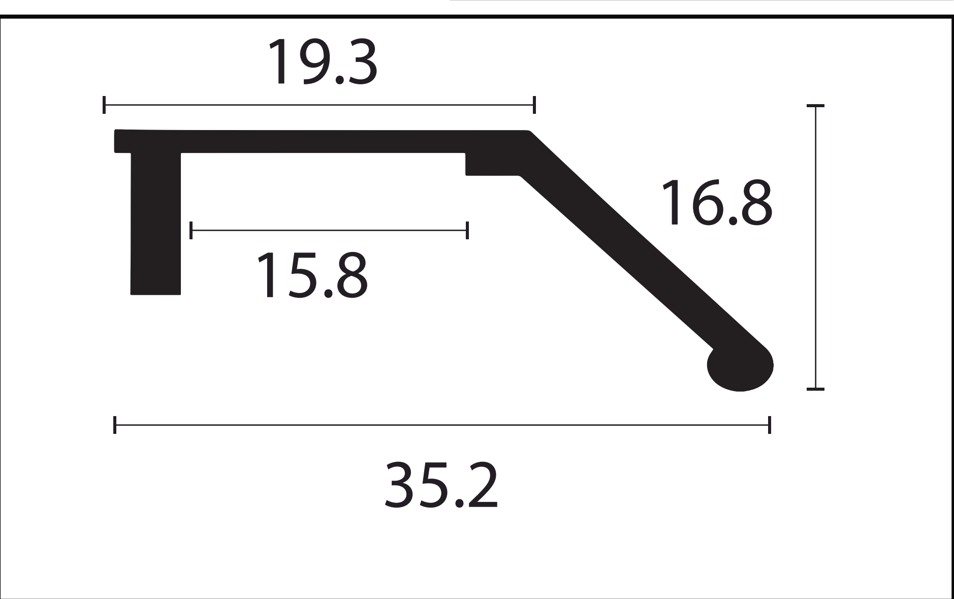
PUXADOR GAP - 9553
