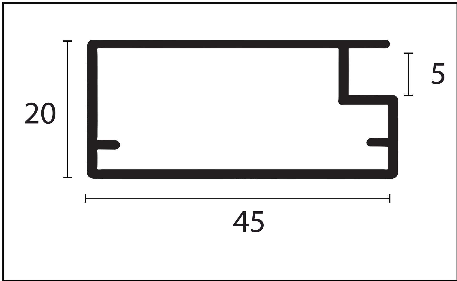
MONTANTE GAP - 1202
