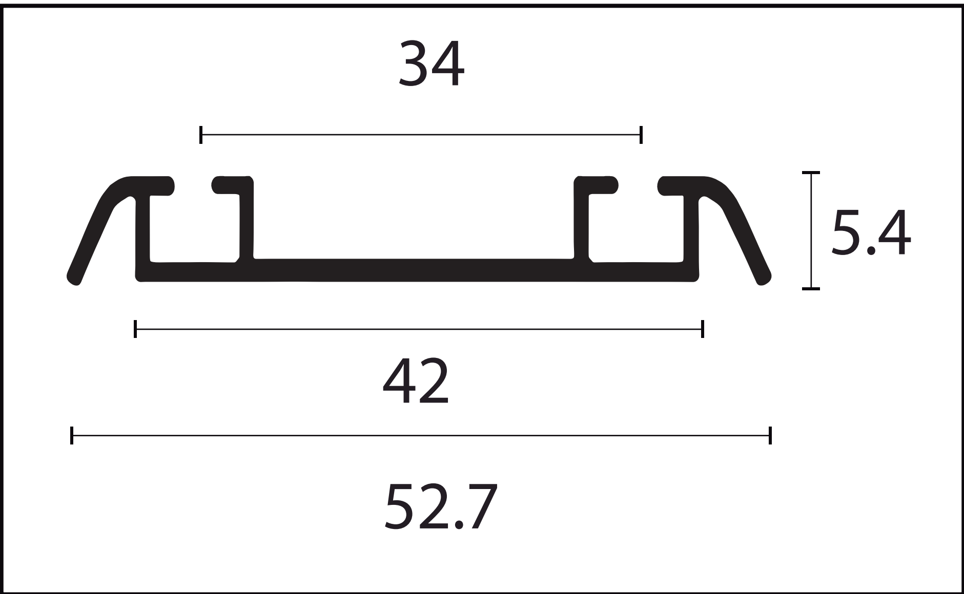
TRILHO GAP - 9014A
