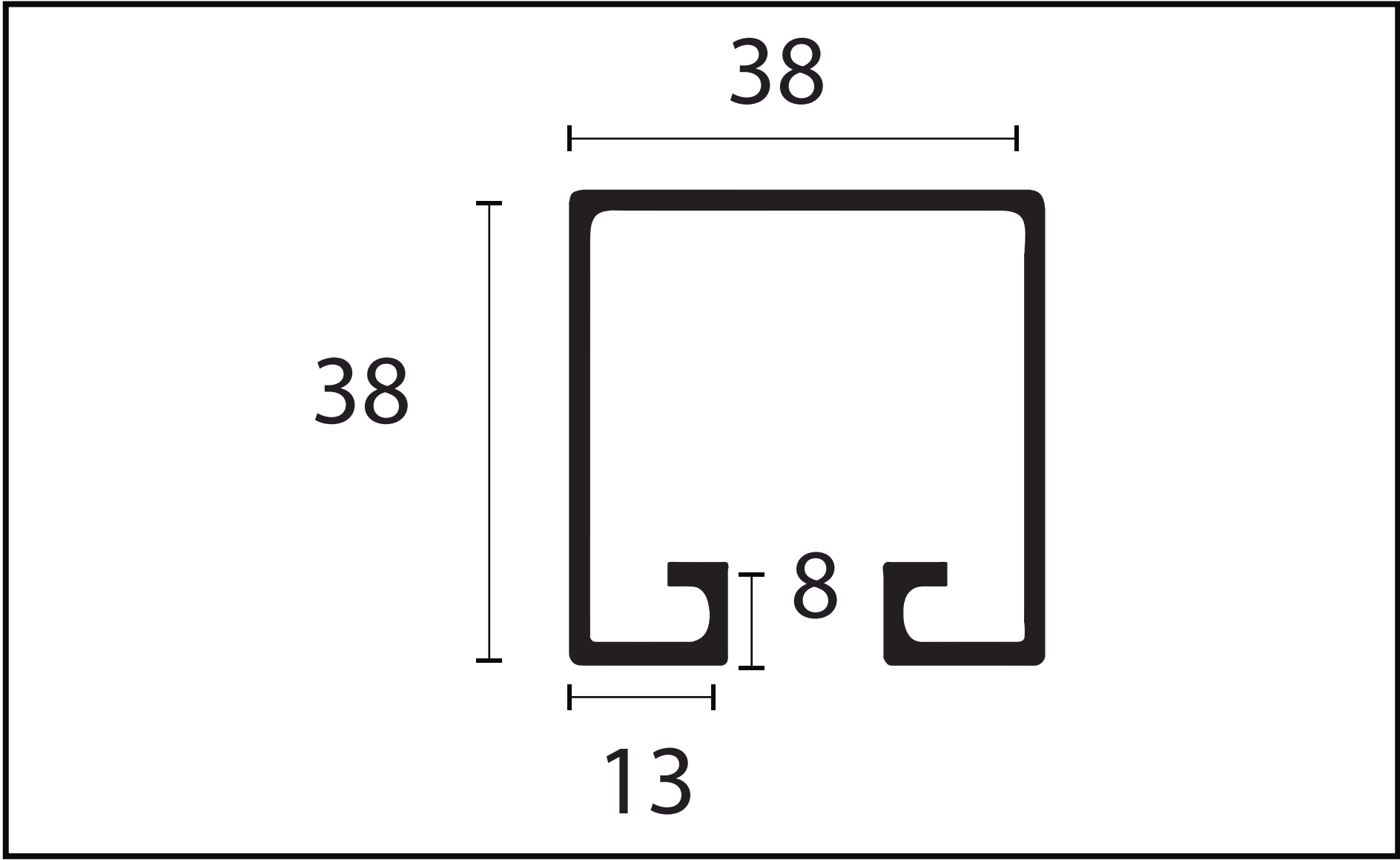
TRILHO GAP - 9919
