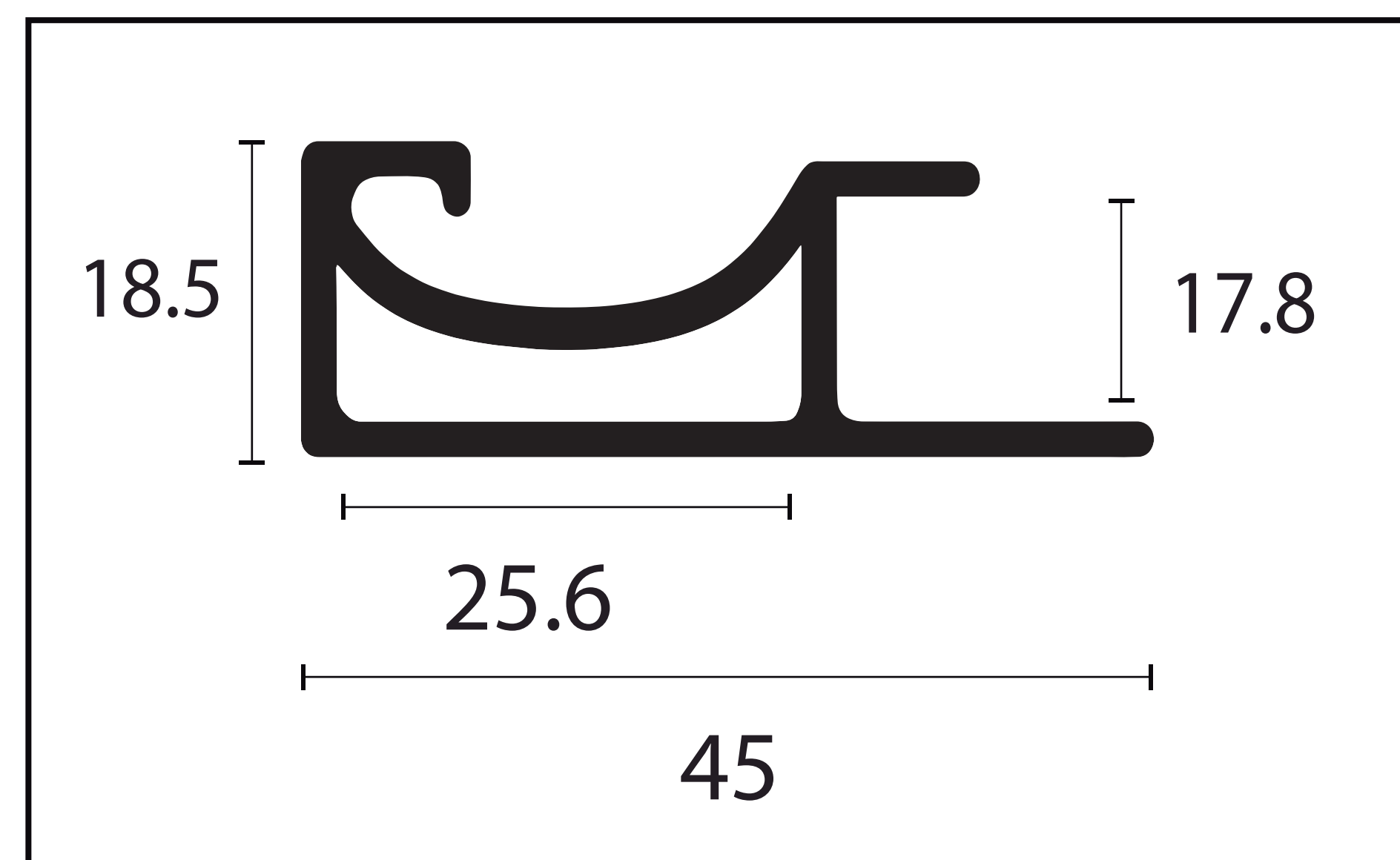
MONTANTE GAP - 1181
