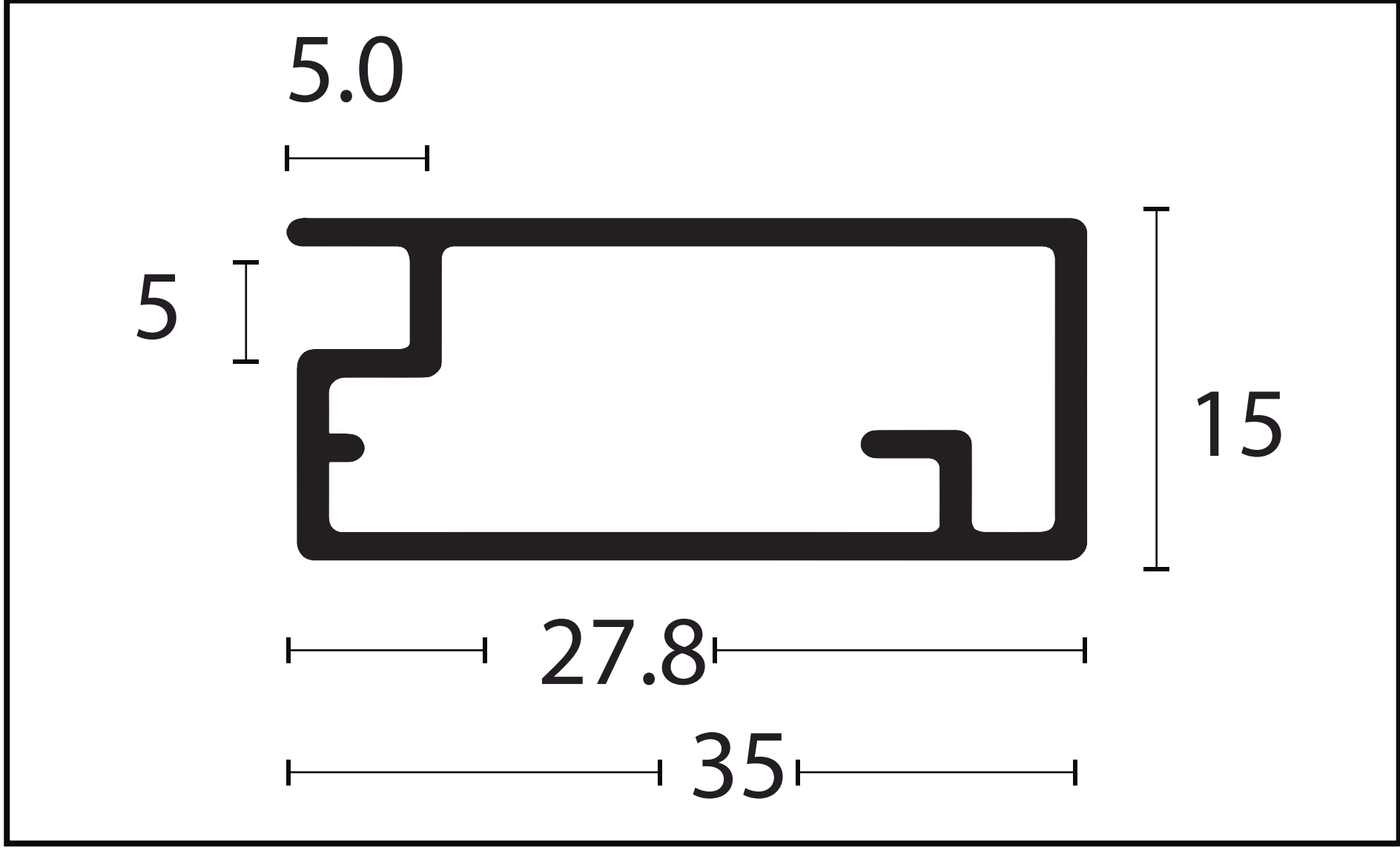
MONTANTE GAP - 996
