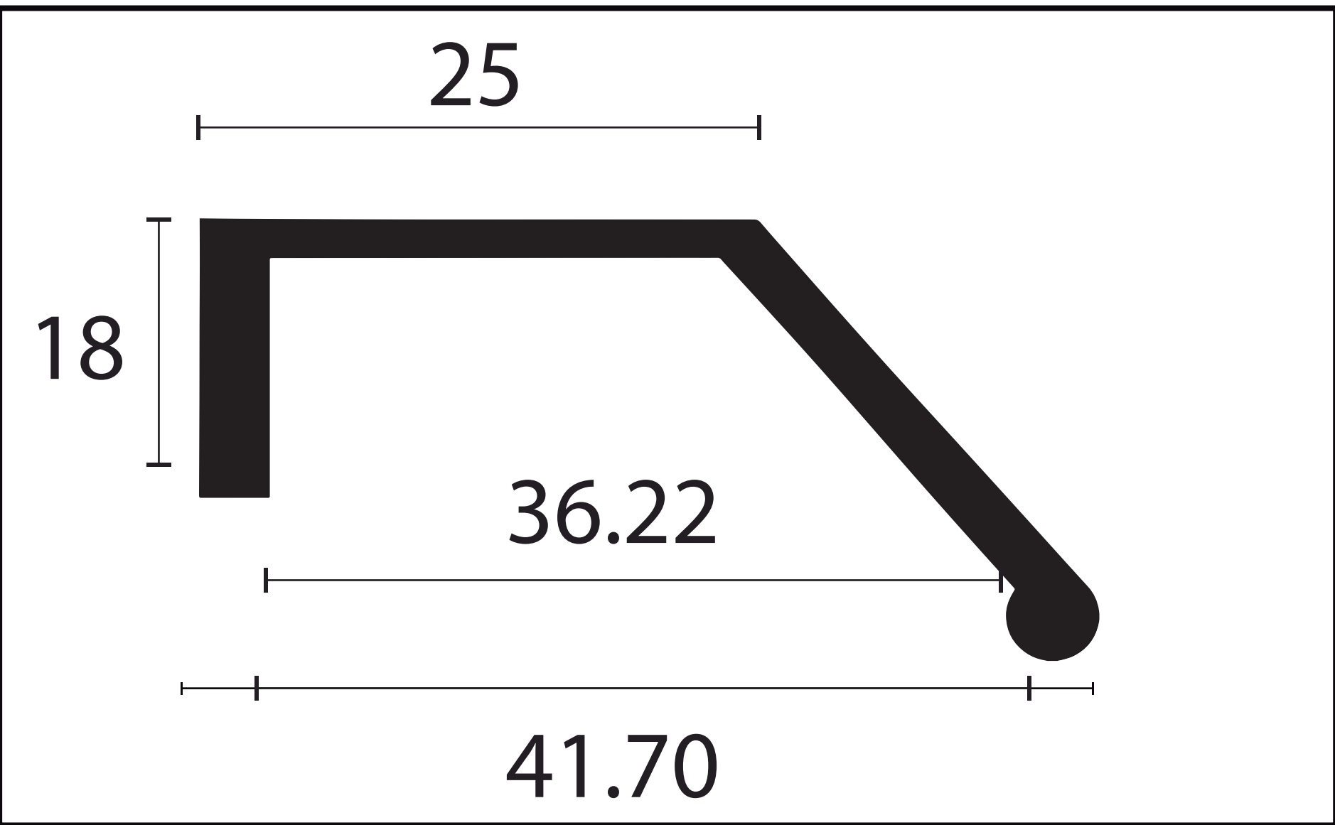
PUXADOR GAP - 9064
