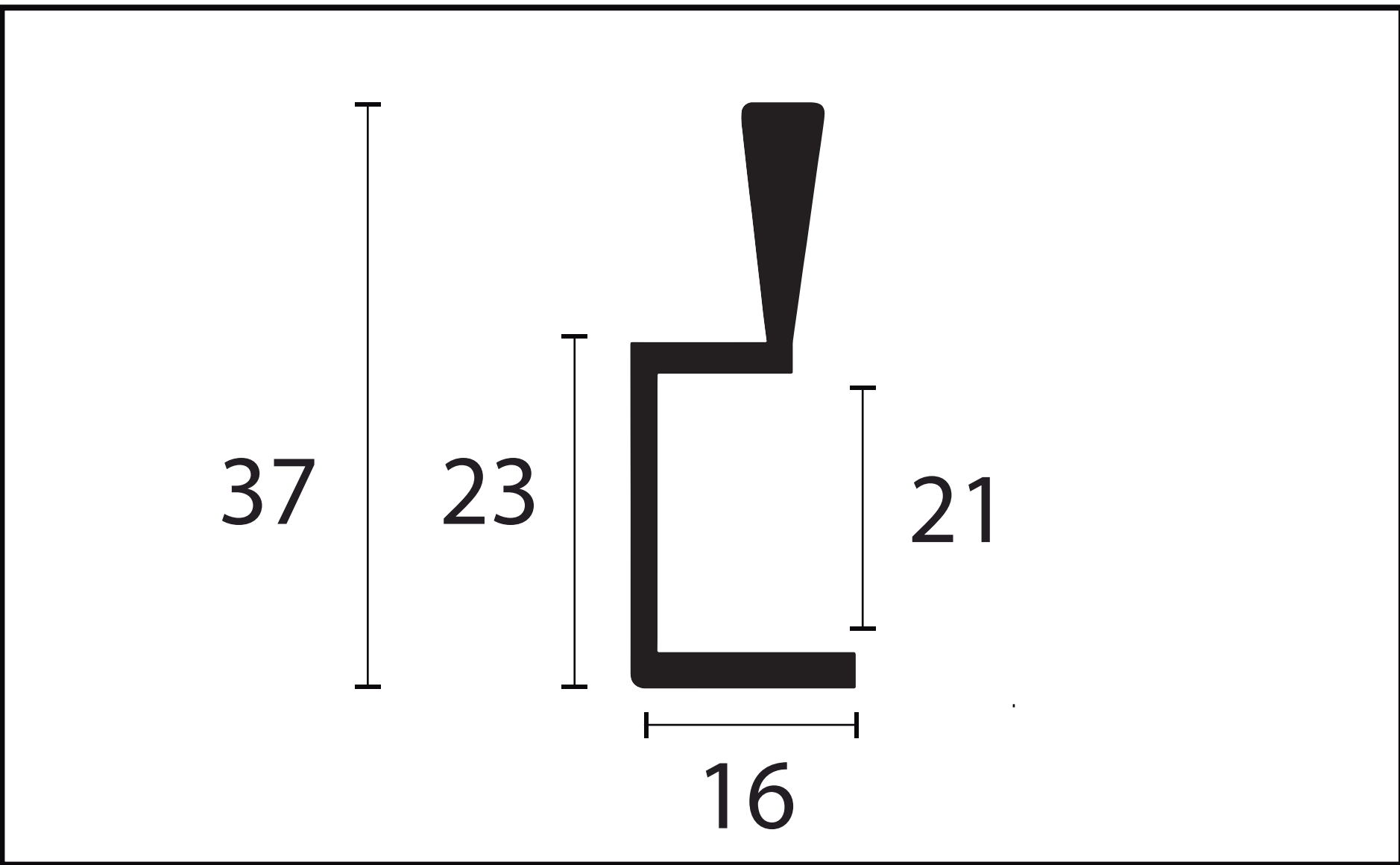
PUXADOR GAP - 9134
