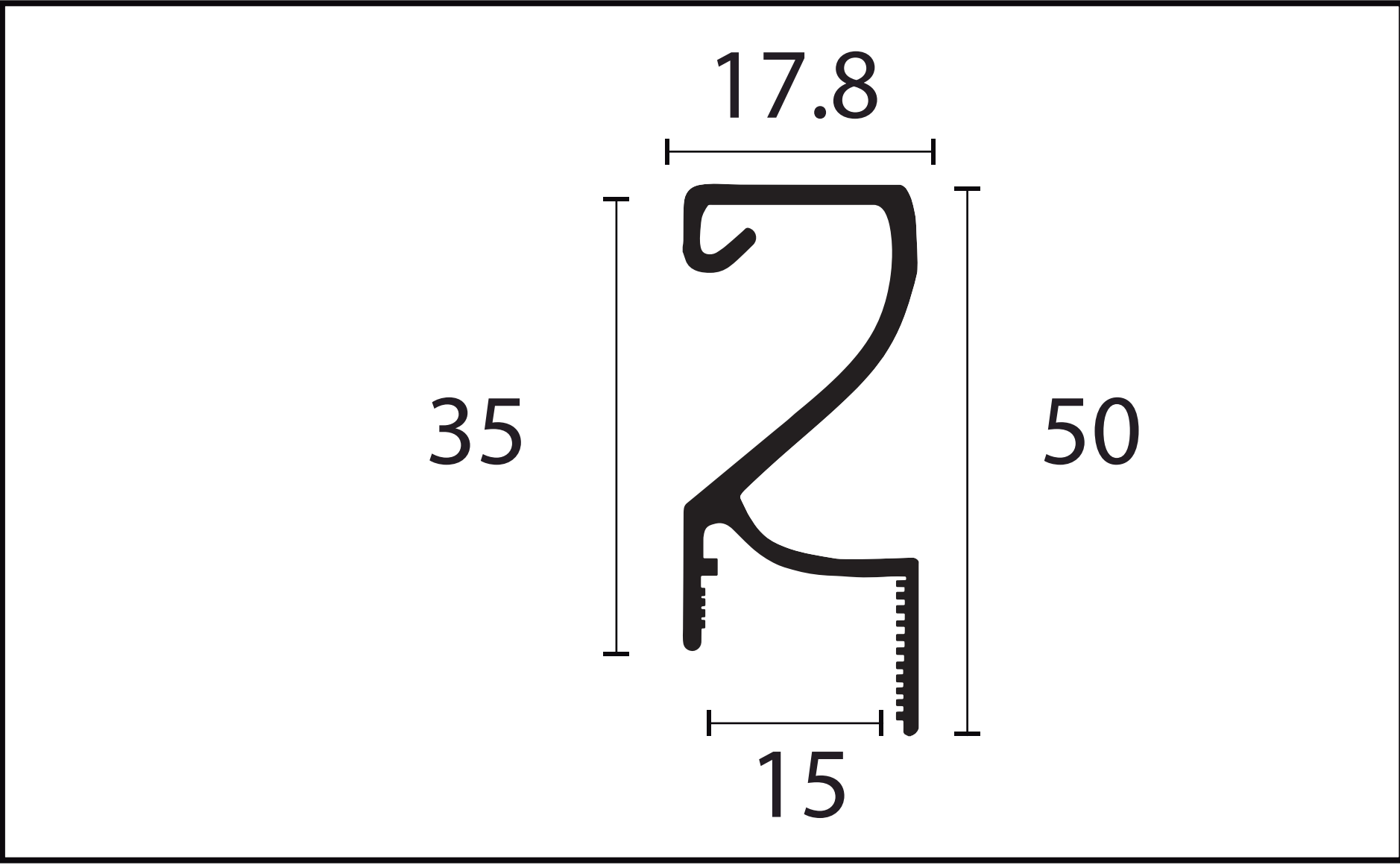
PUXADOR GAP - 9133L
