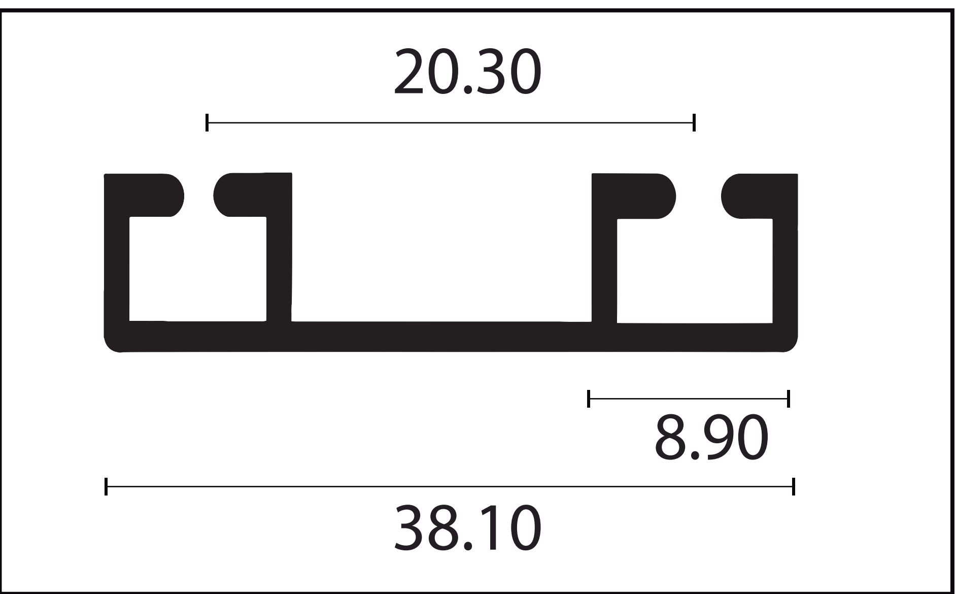
TRILHO GAP - 9013B
