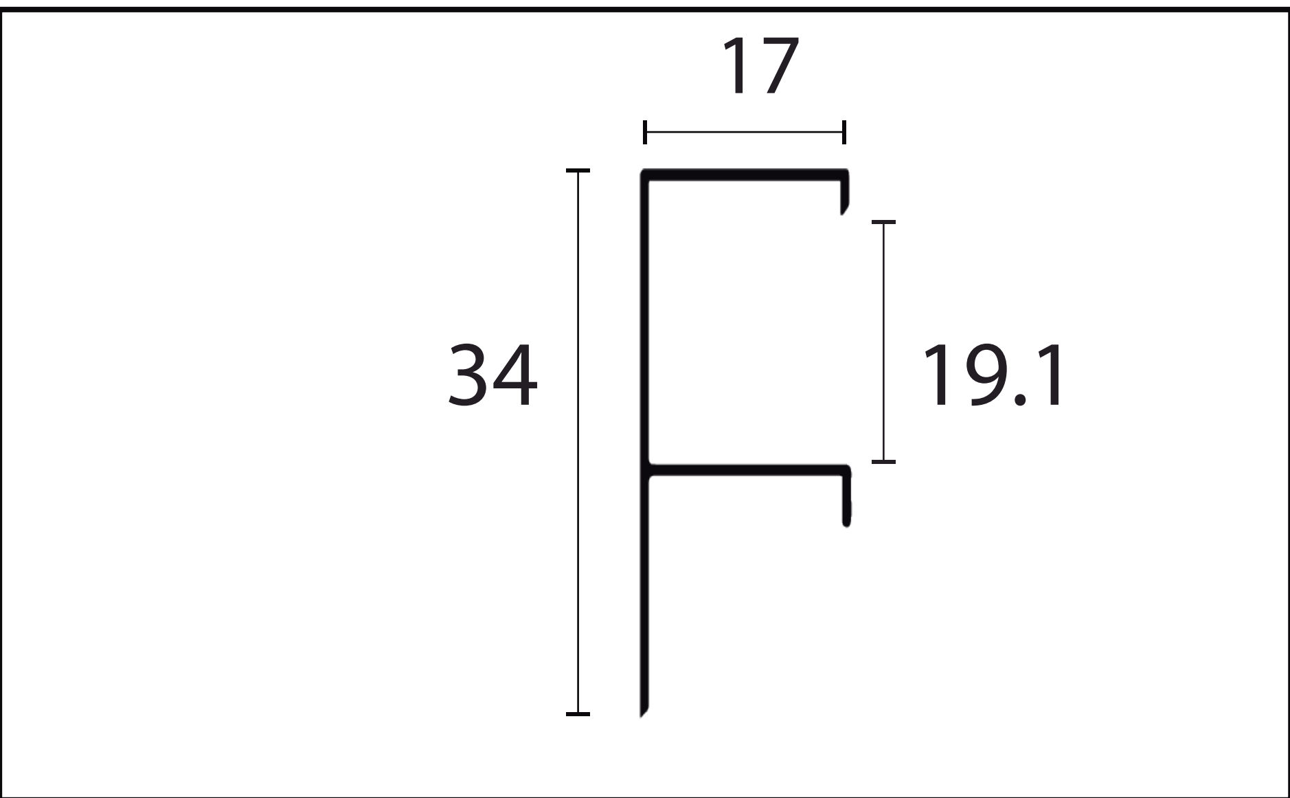
PUXADOR GAP - 9479
