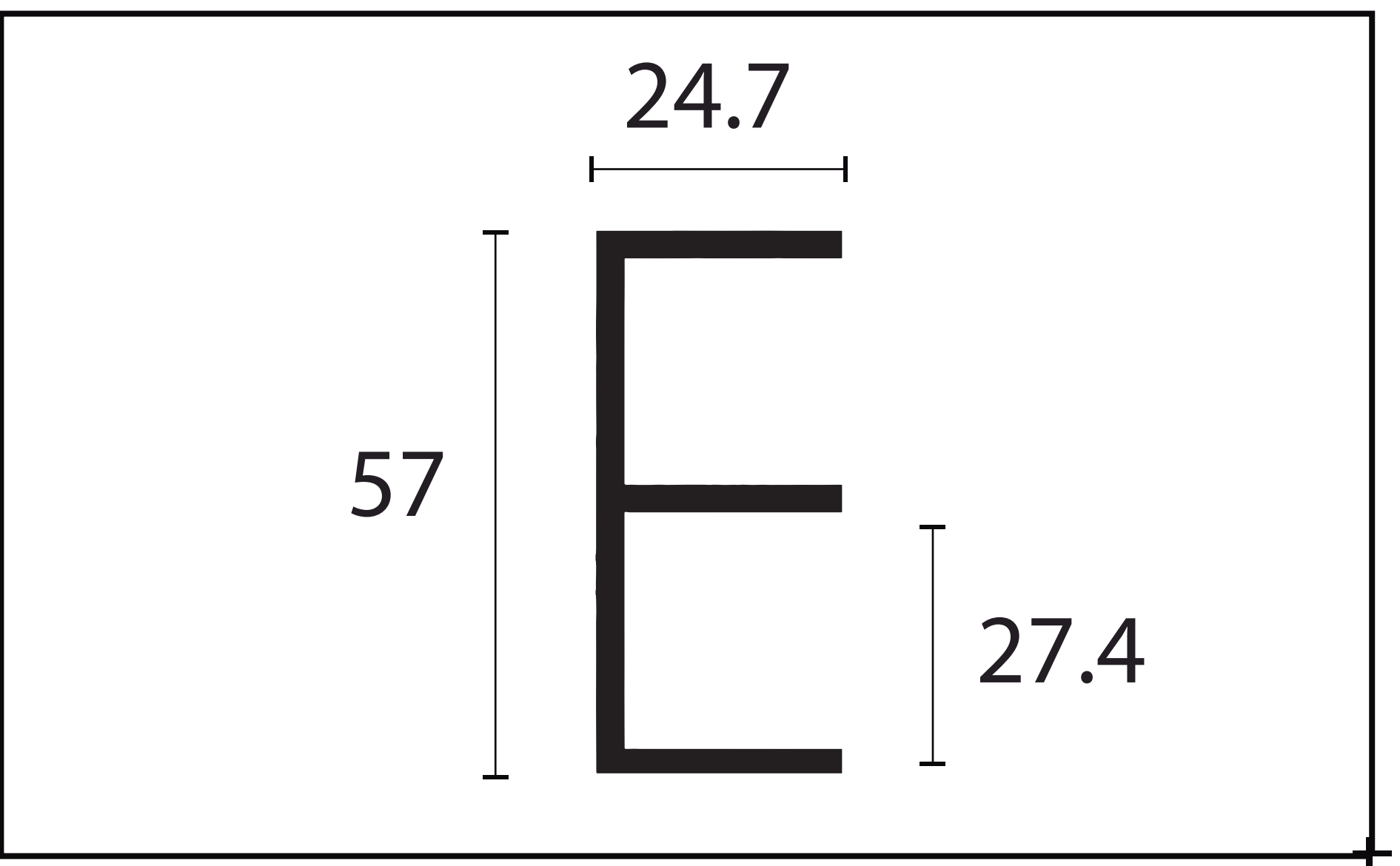
TRILHO GAP - 6363
