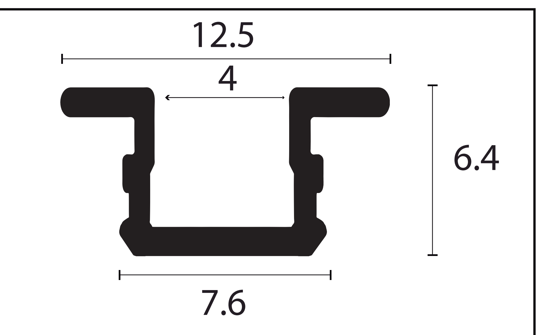
TRILHO GAP - 9848
