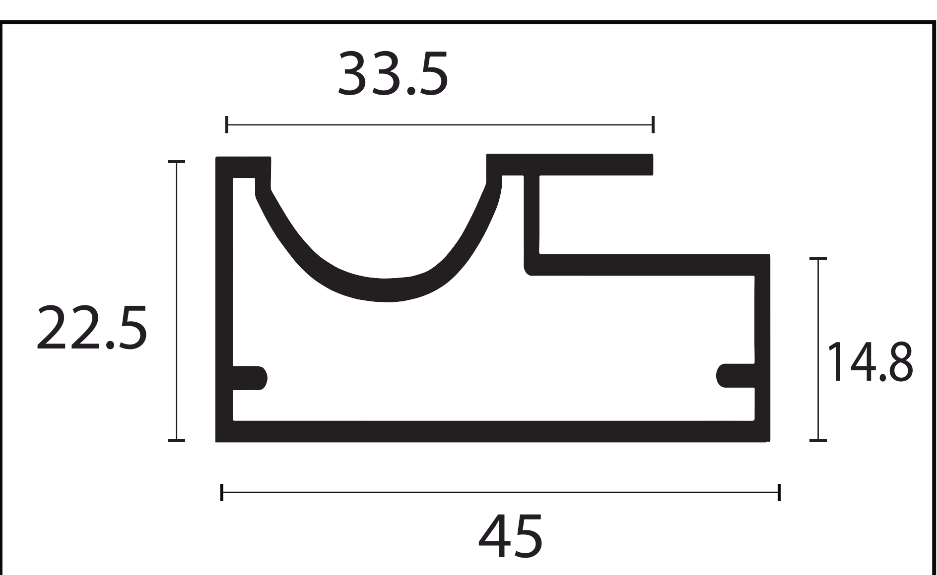
MONTANTE GAP - 617
