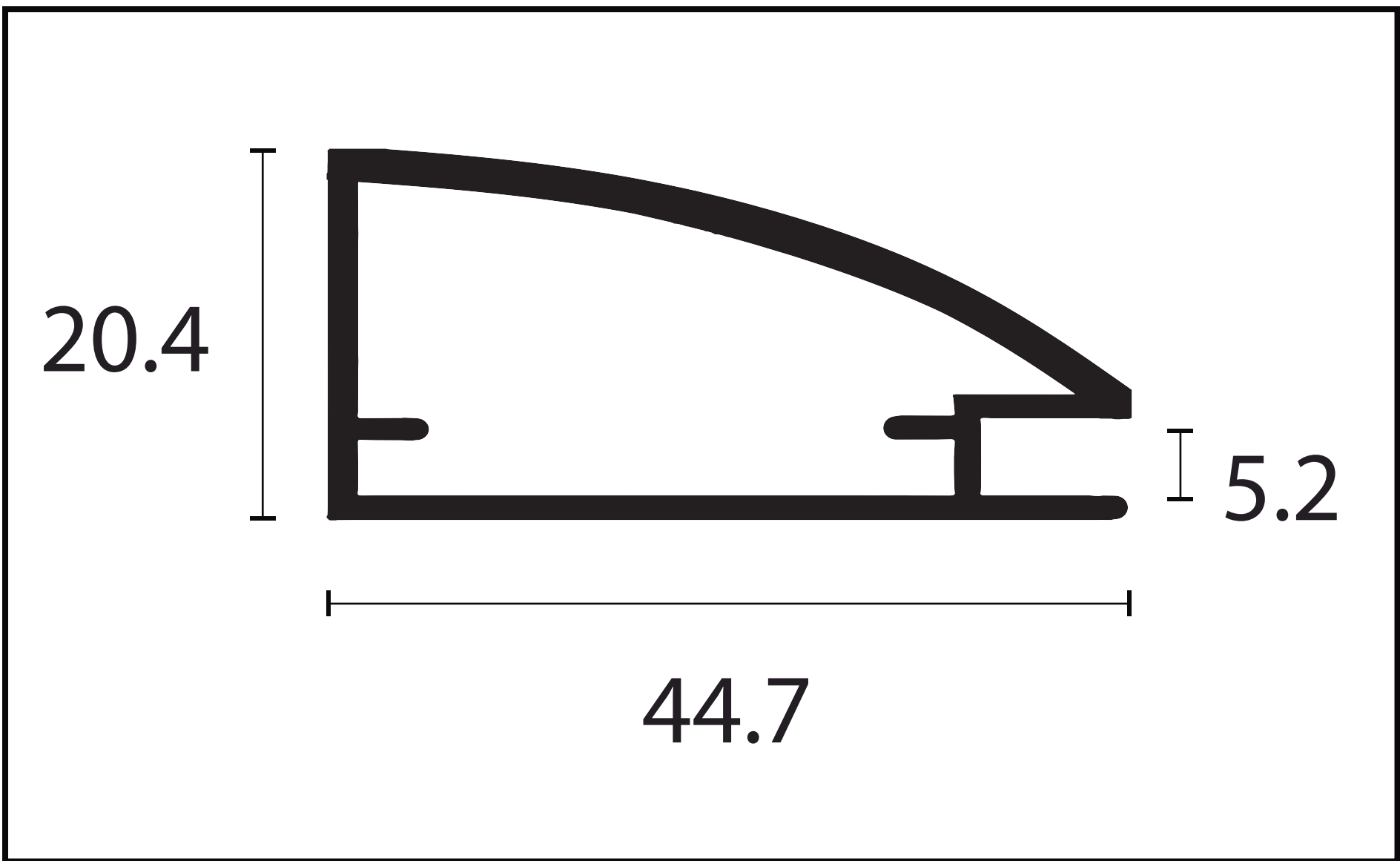
MONTANTE GAP - 9528E
