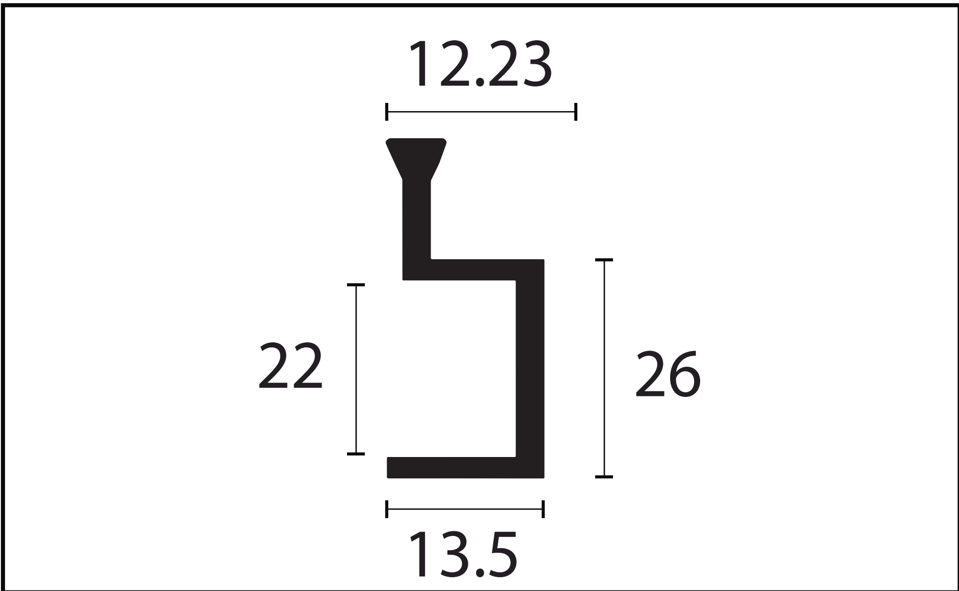
PUXADOR GAP - 9133
