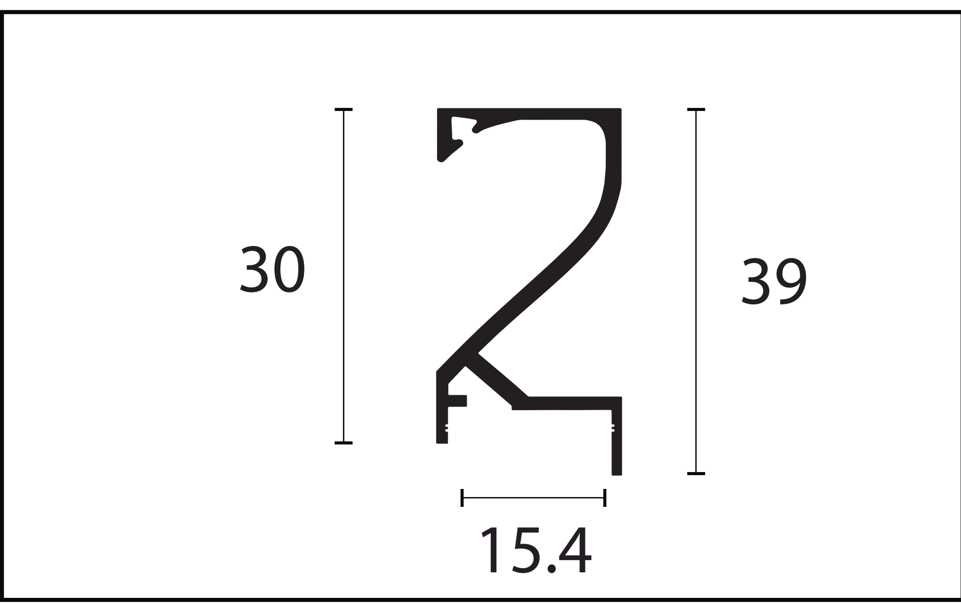
PUXADOR GAP - 946L
