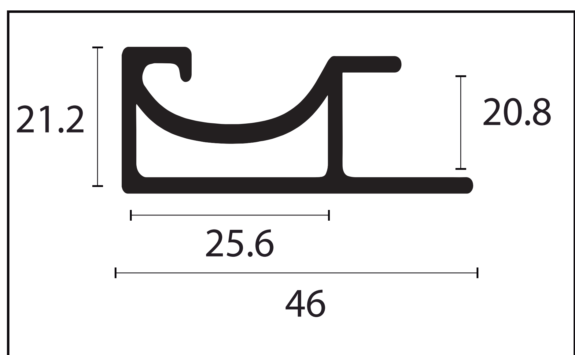
MONTANTE GAP - 616
