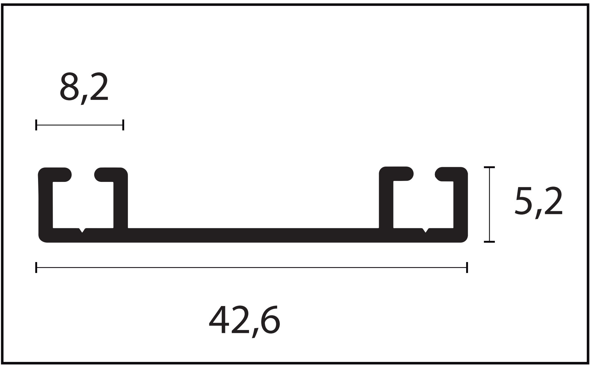
TRILHO GAP - 9013L
