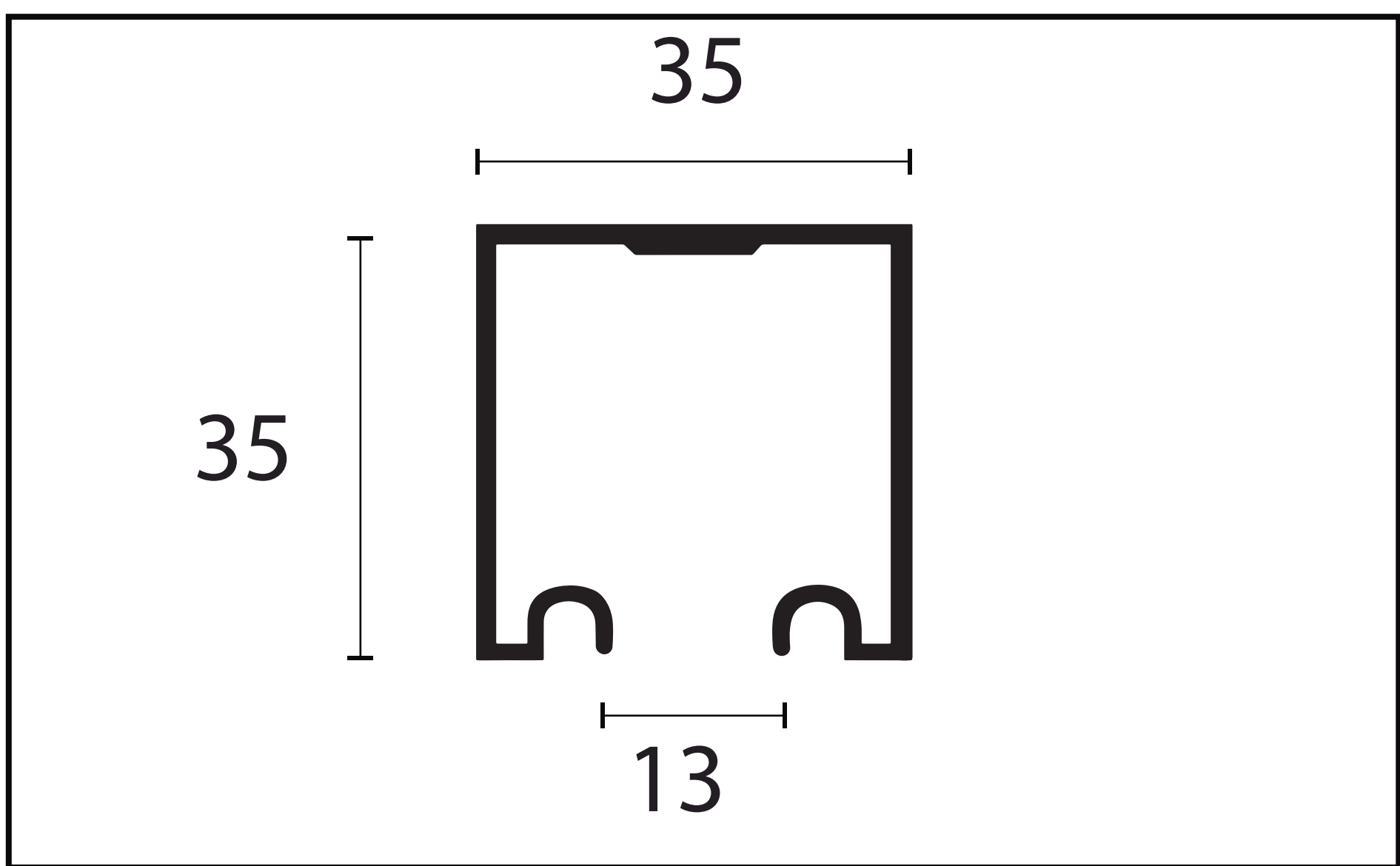
TRILHO GAP - 9918
