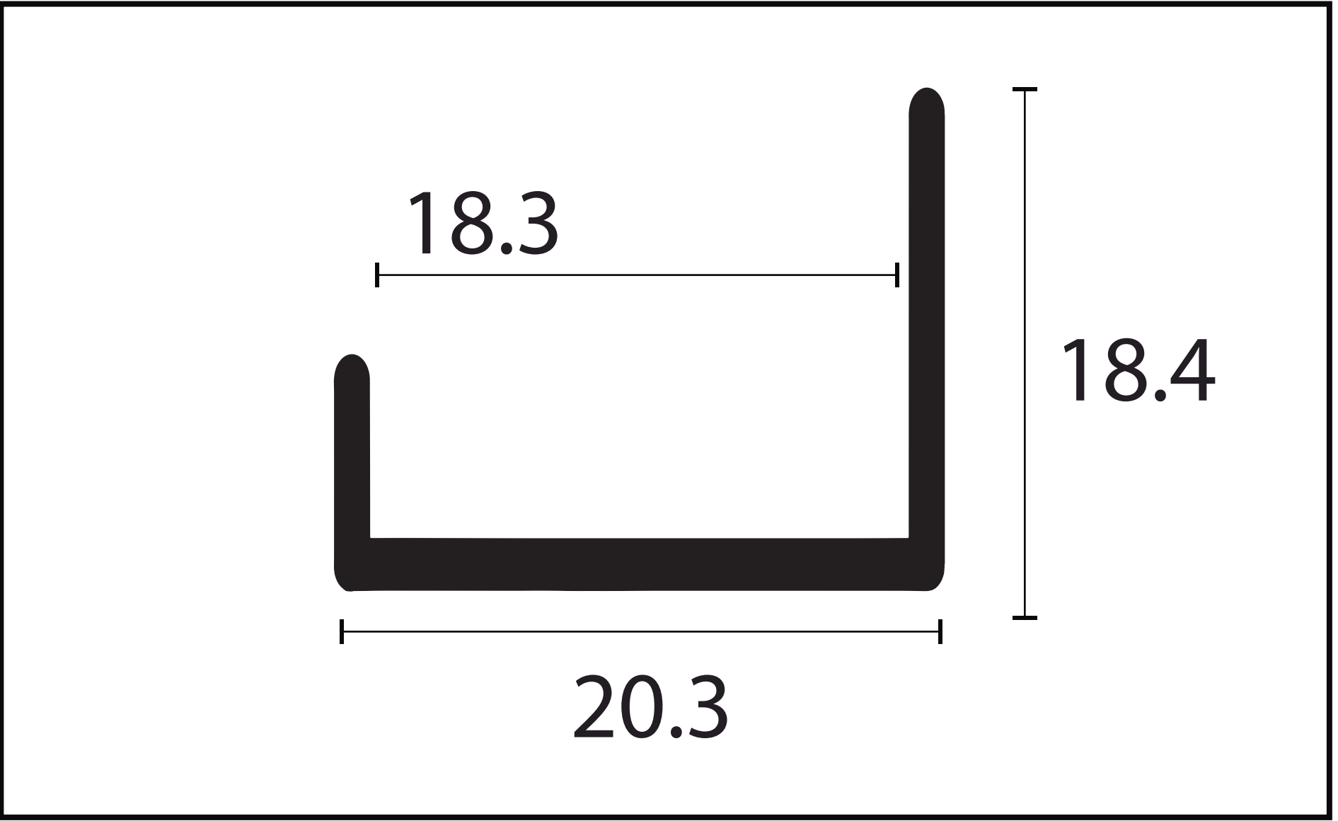
TRILHO GAP - 9198
