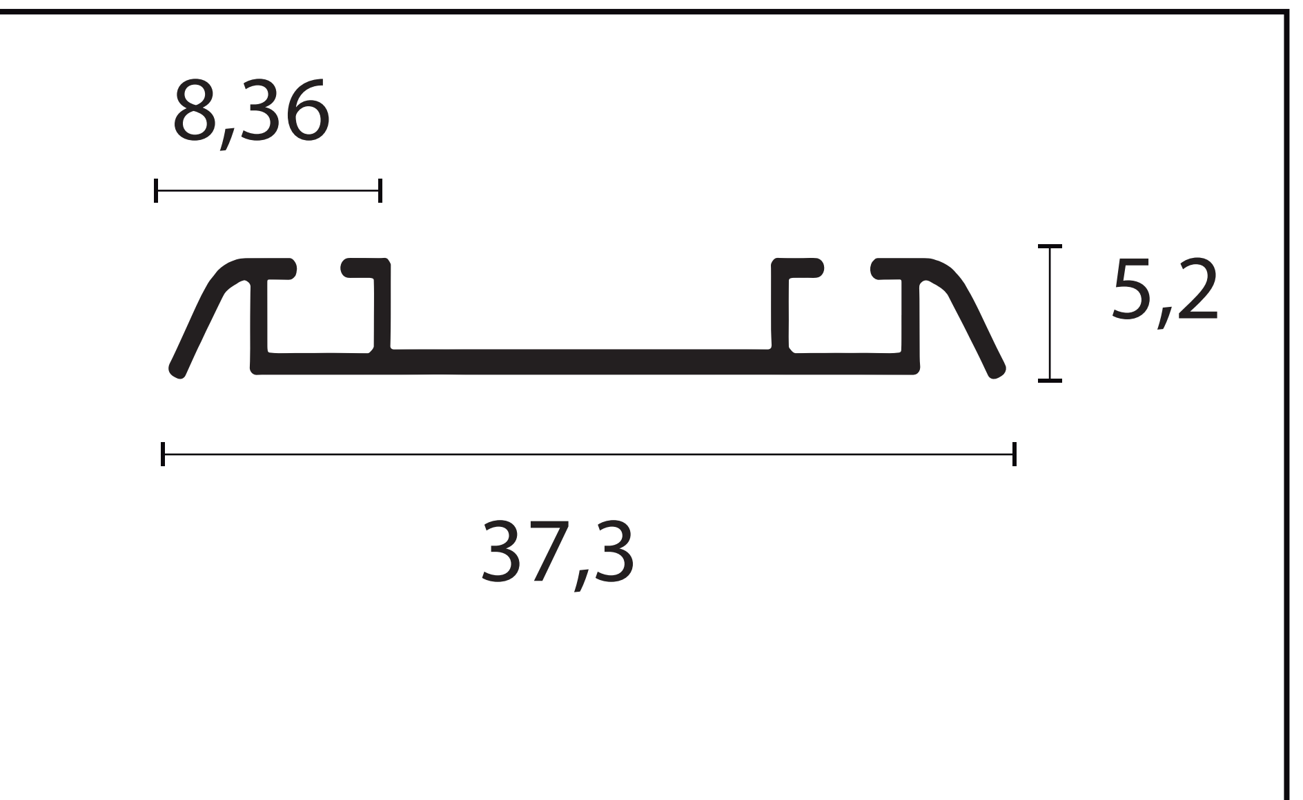
TRILHO GAP - 9014L
