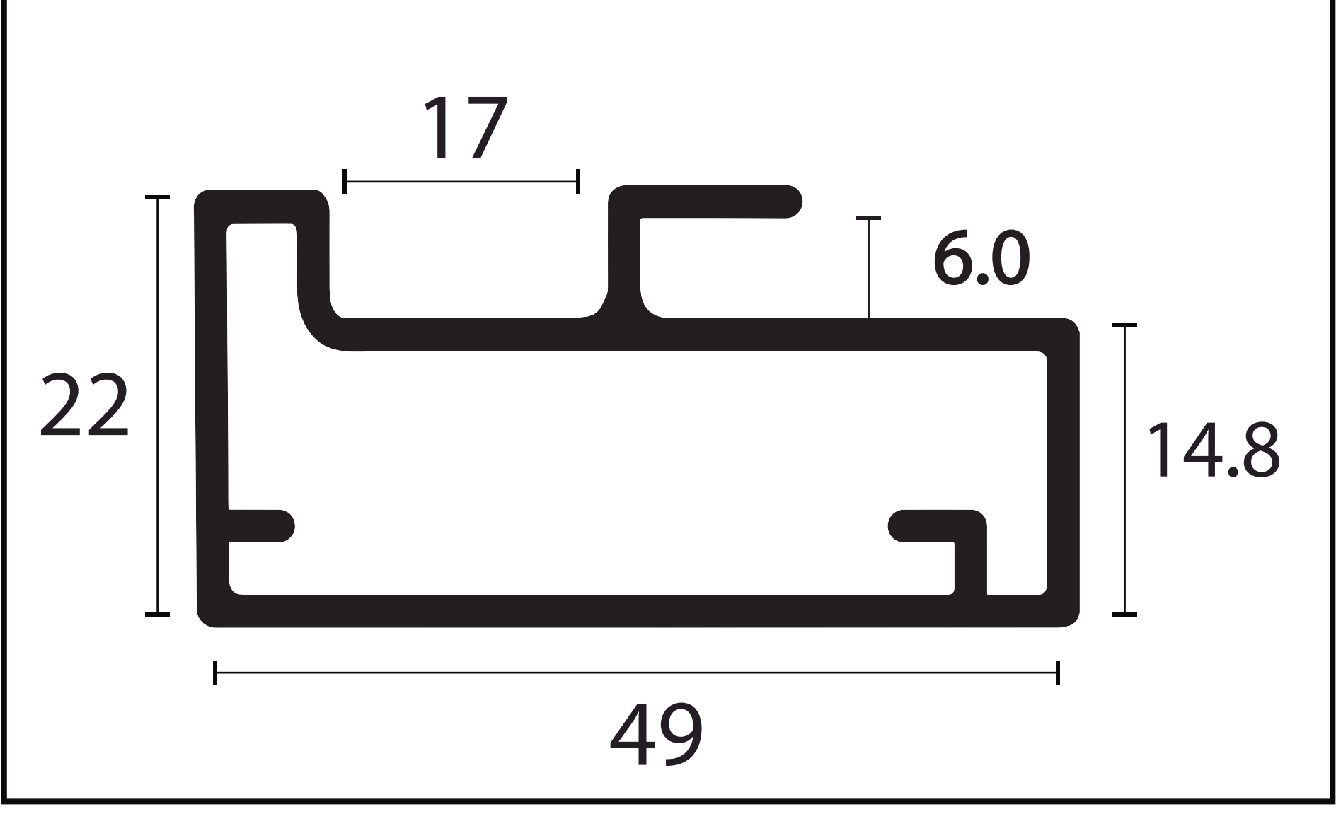
MONTANTE GAP - 1490
