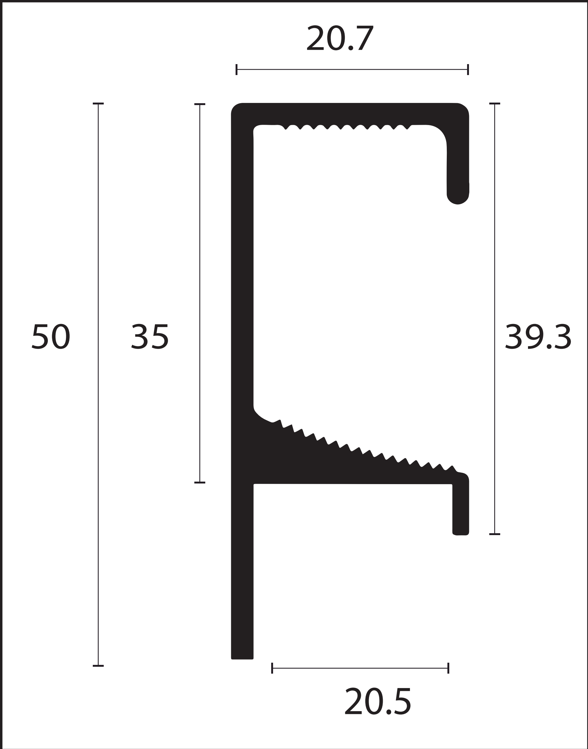
PUXADOR GAP - 9000
