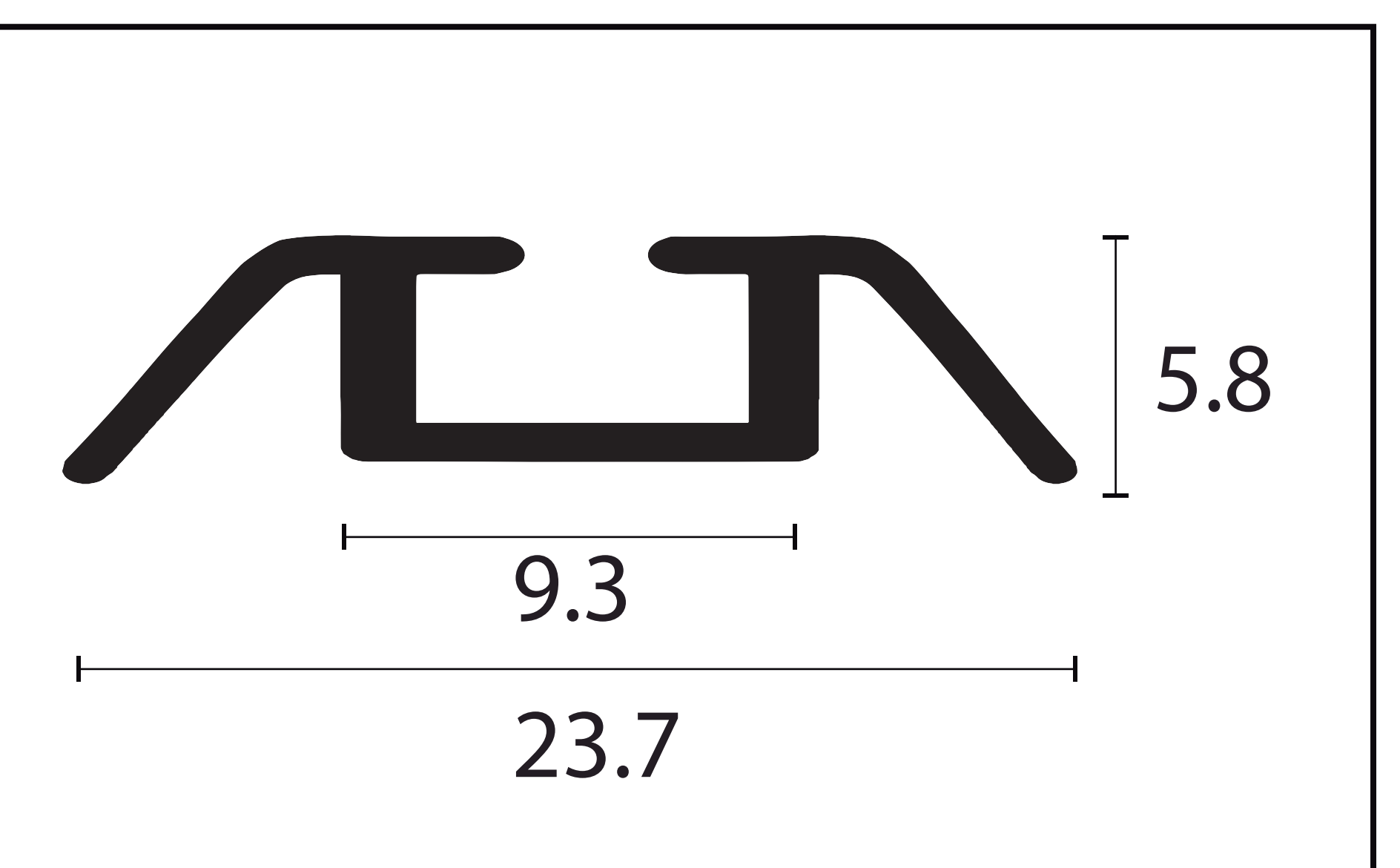
TUBO GAP - 003
