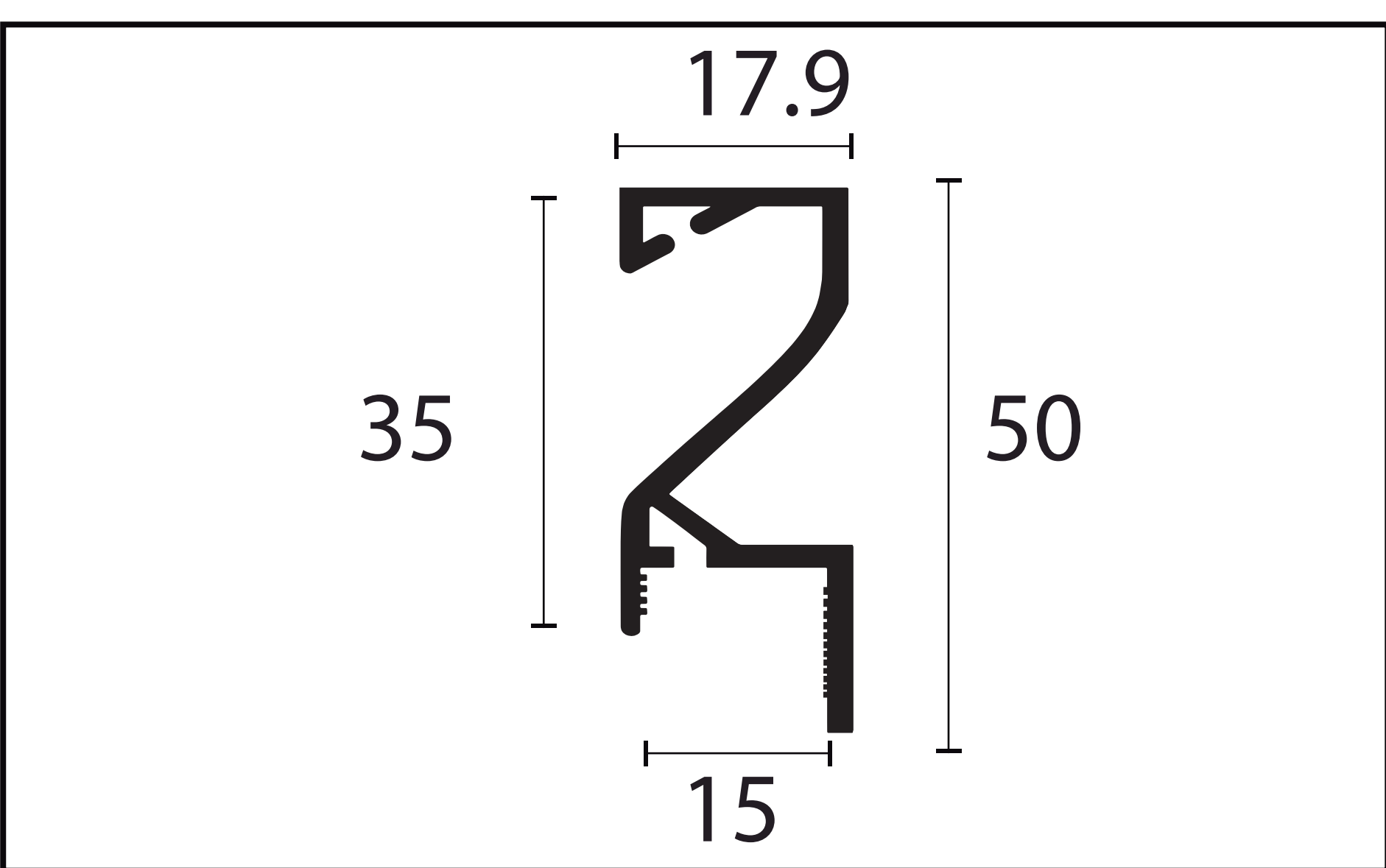
PUXADOR GAP - 9134L
