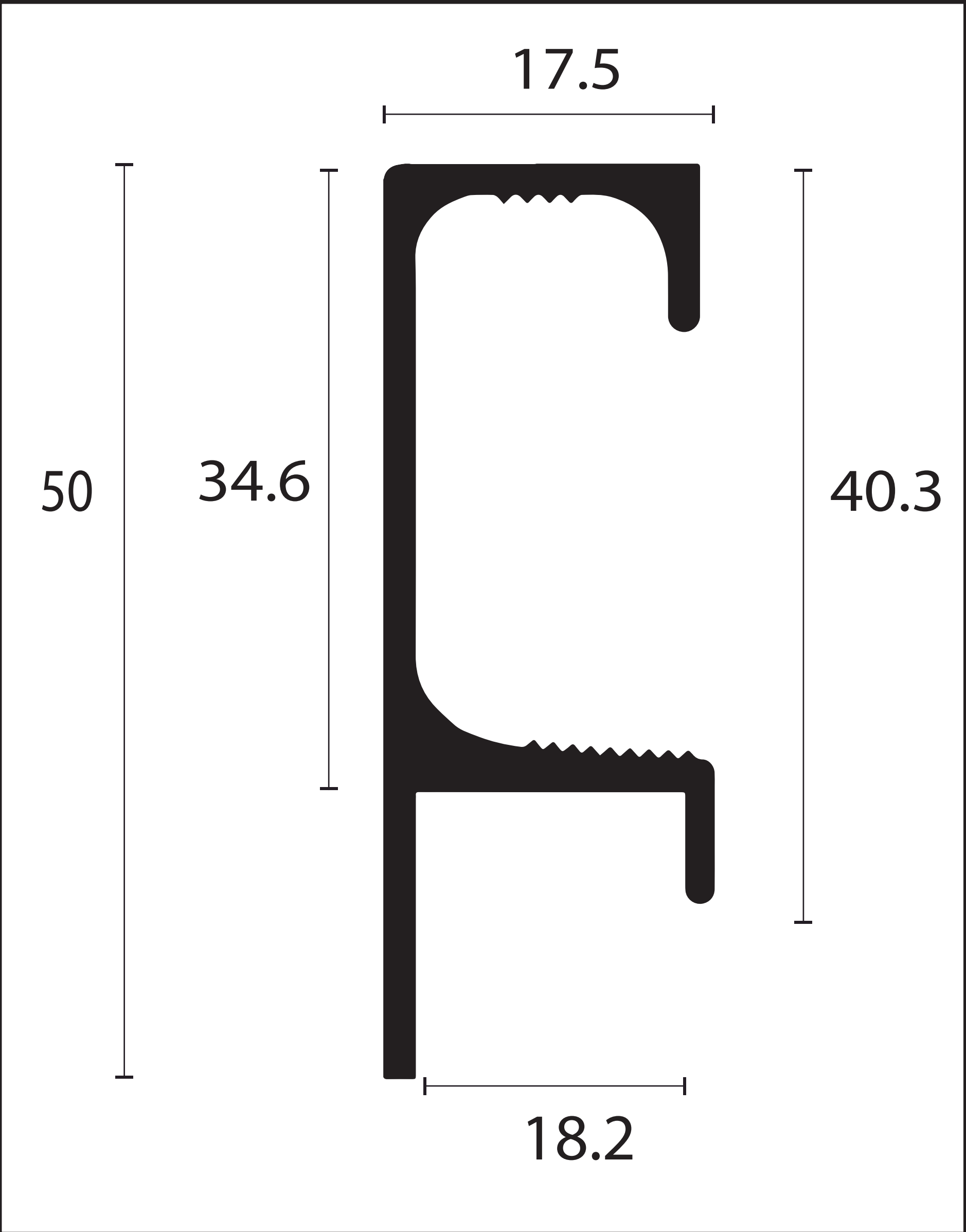
PUXADOR GAP - 9069
