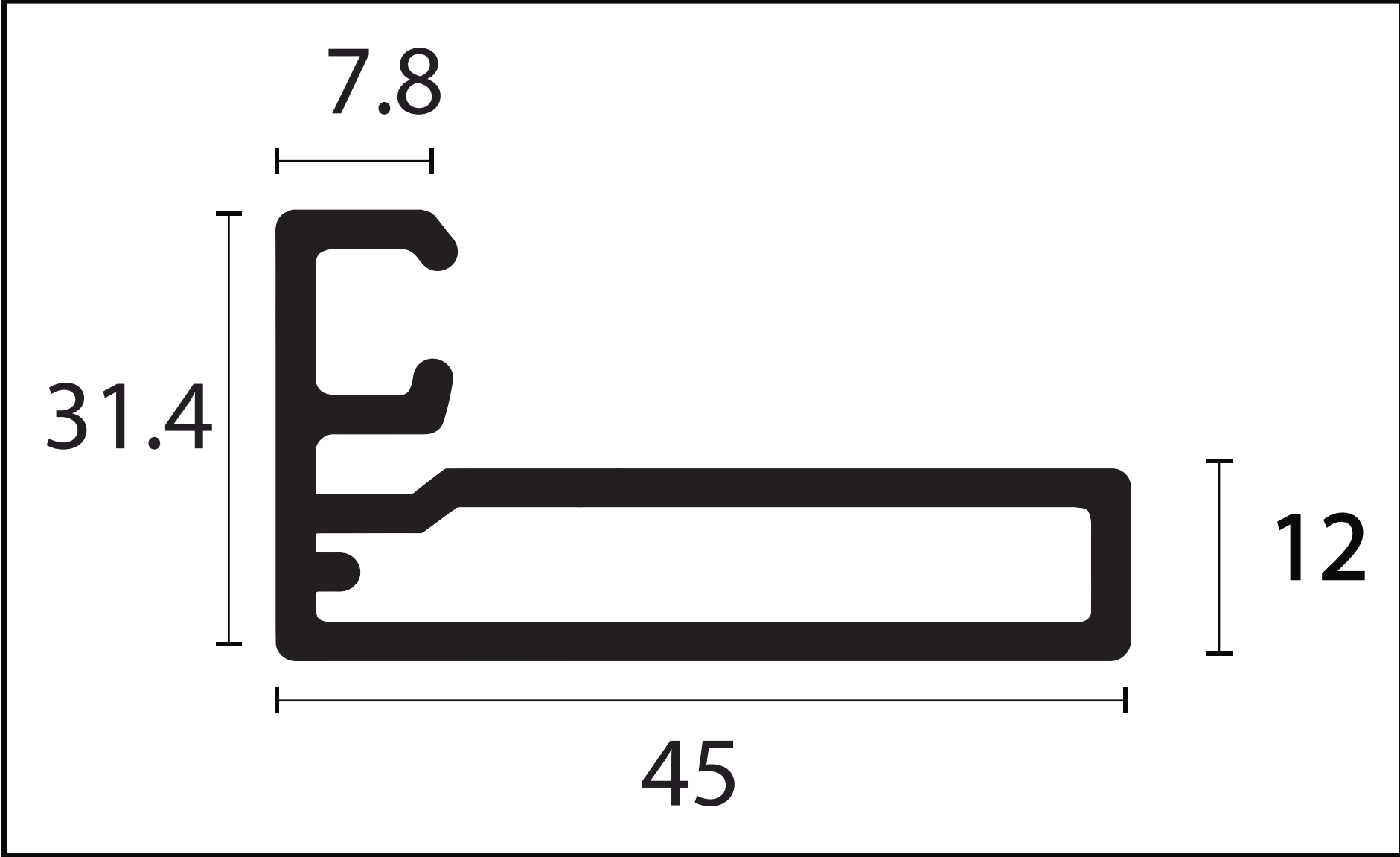
MONTANTE GAP - 995
