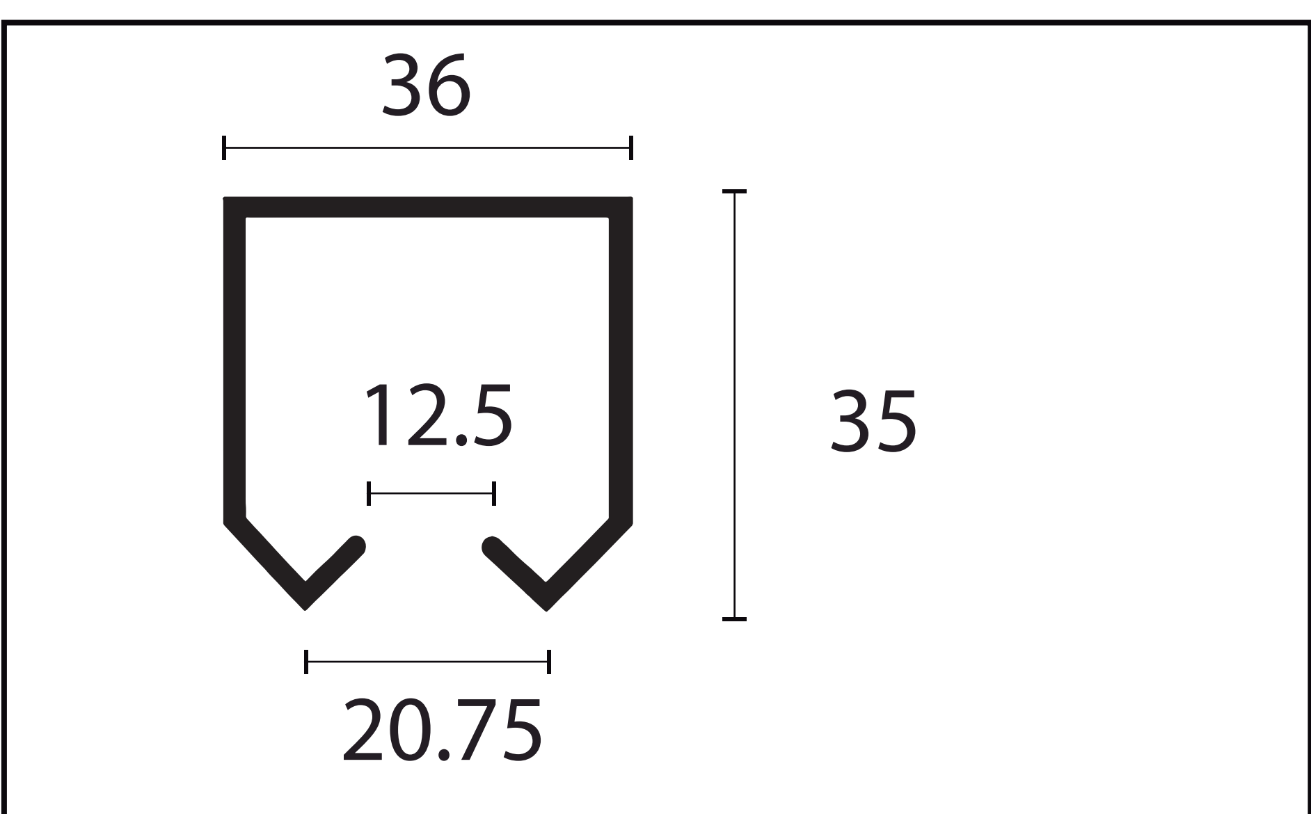
TRILHO GAP - 9030A
