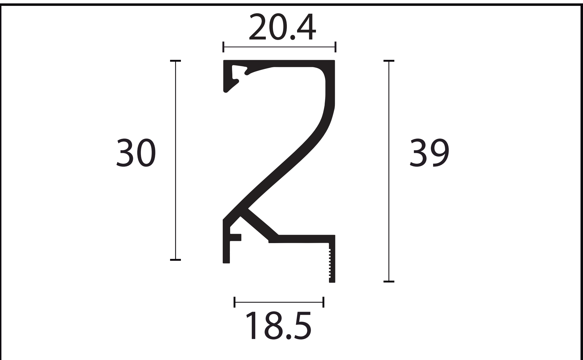
PUXADOR GAP - 47312
