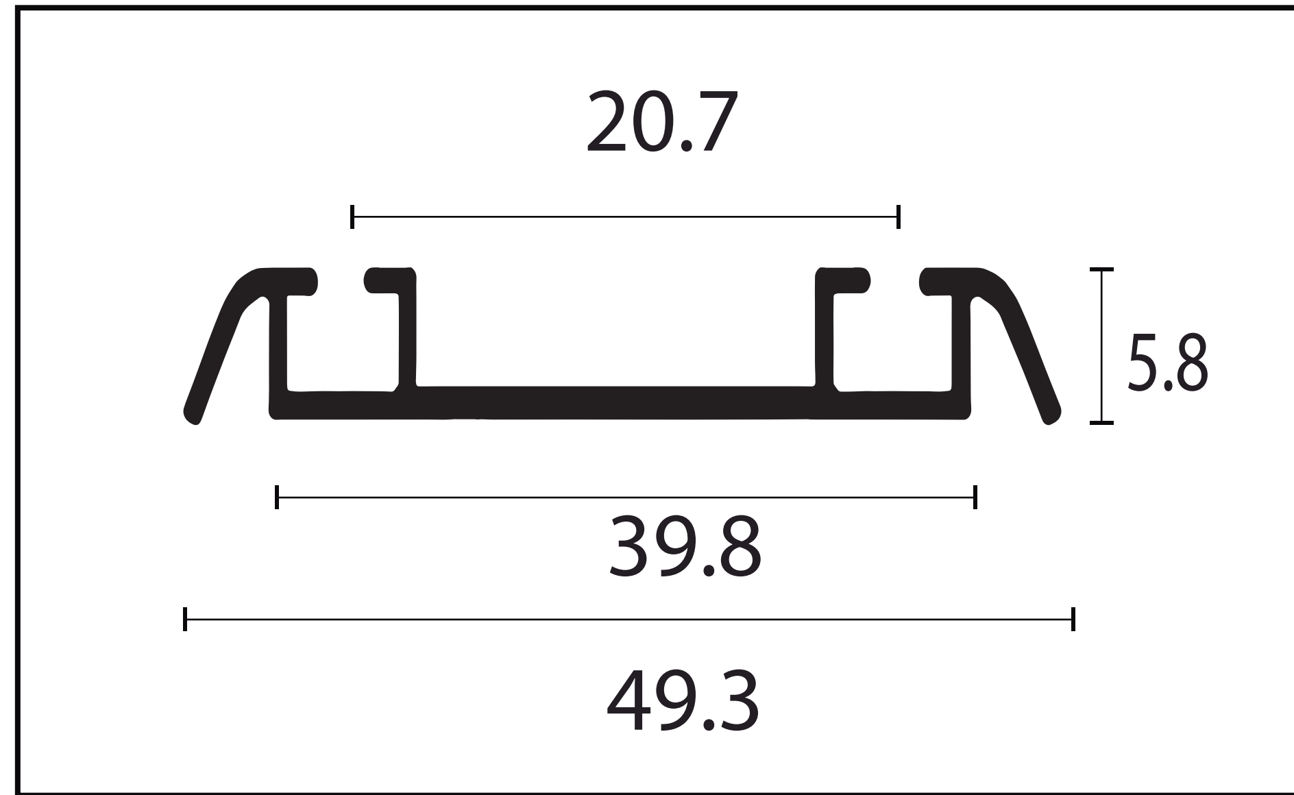
TRILHO GAP - 9014
