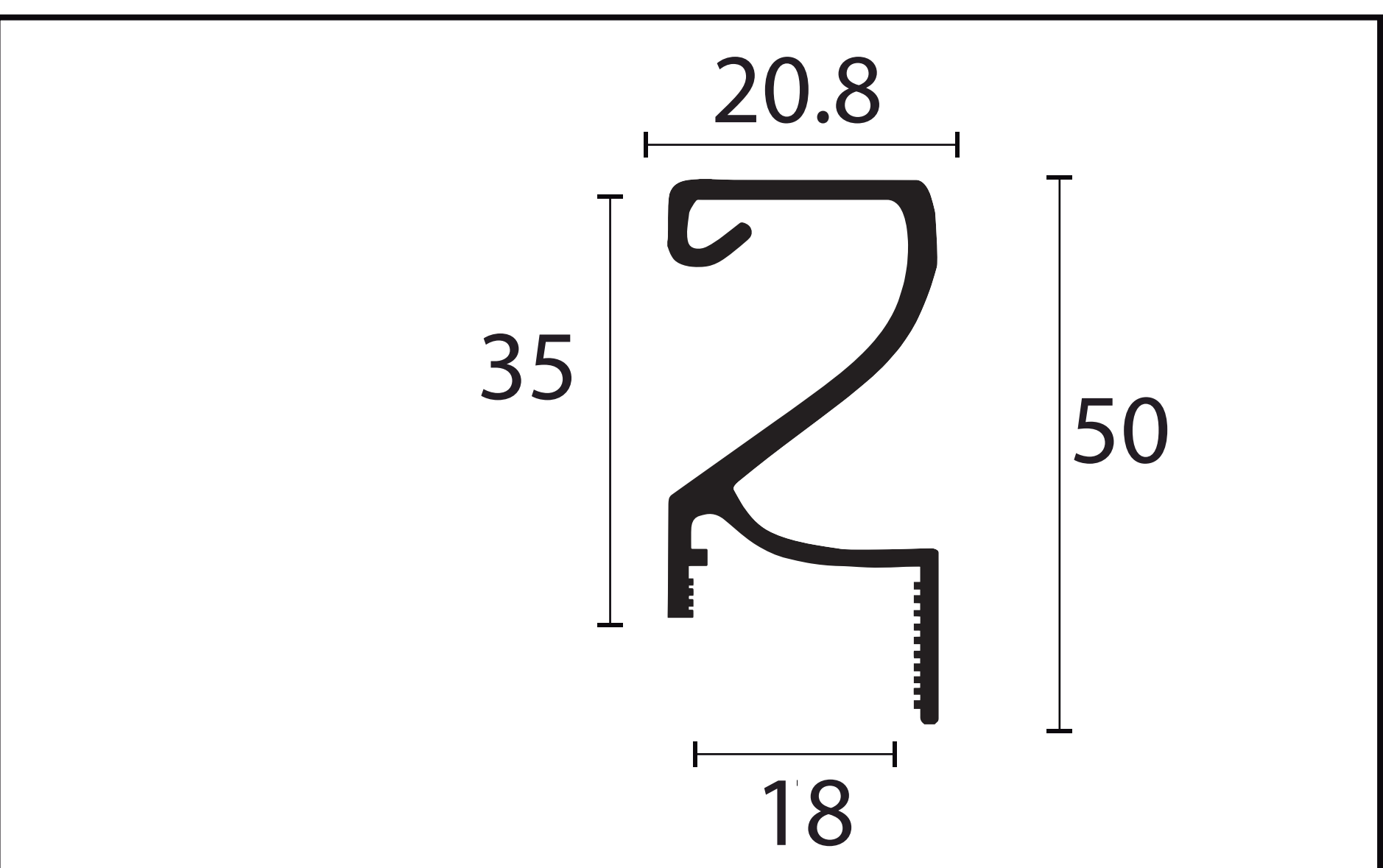
PUXADOR GAP - 46313
