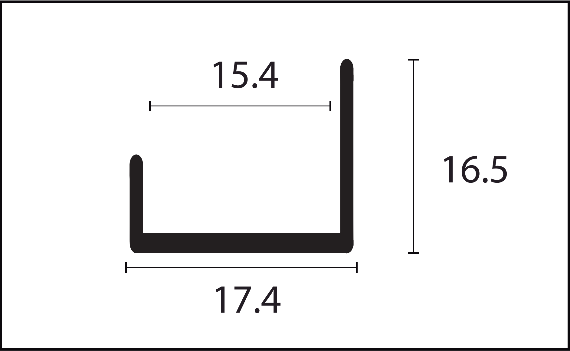
TRILHO GAP - 9915
