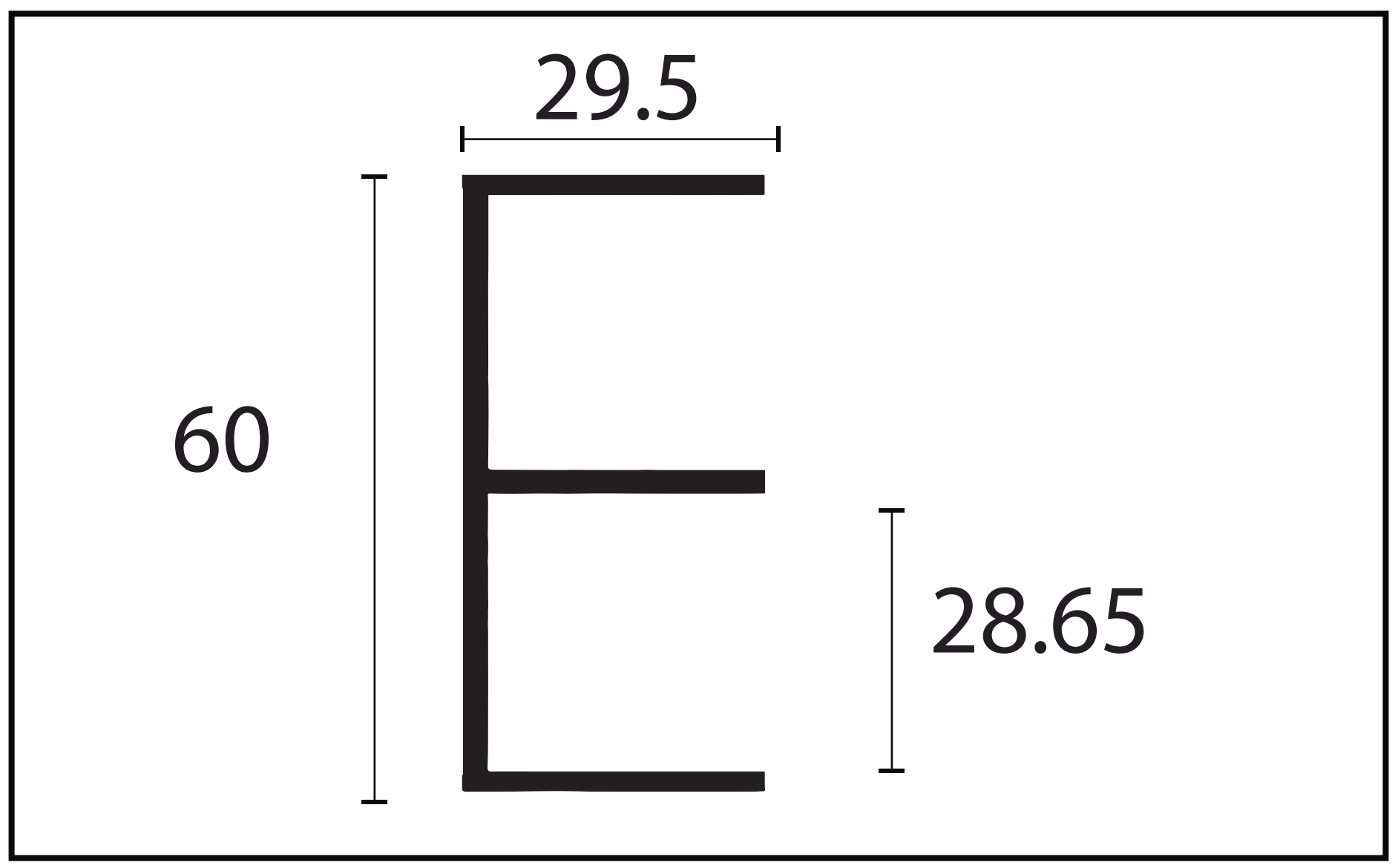
TRILHO GAP - 6262
